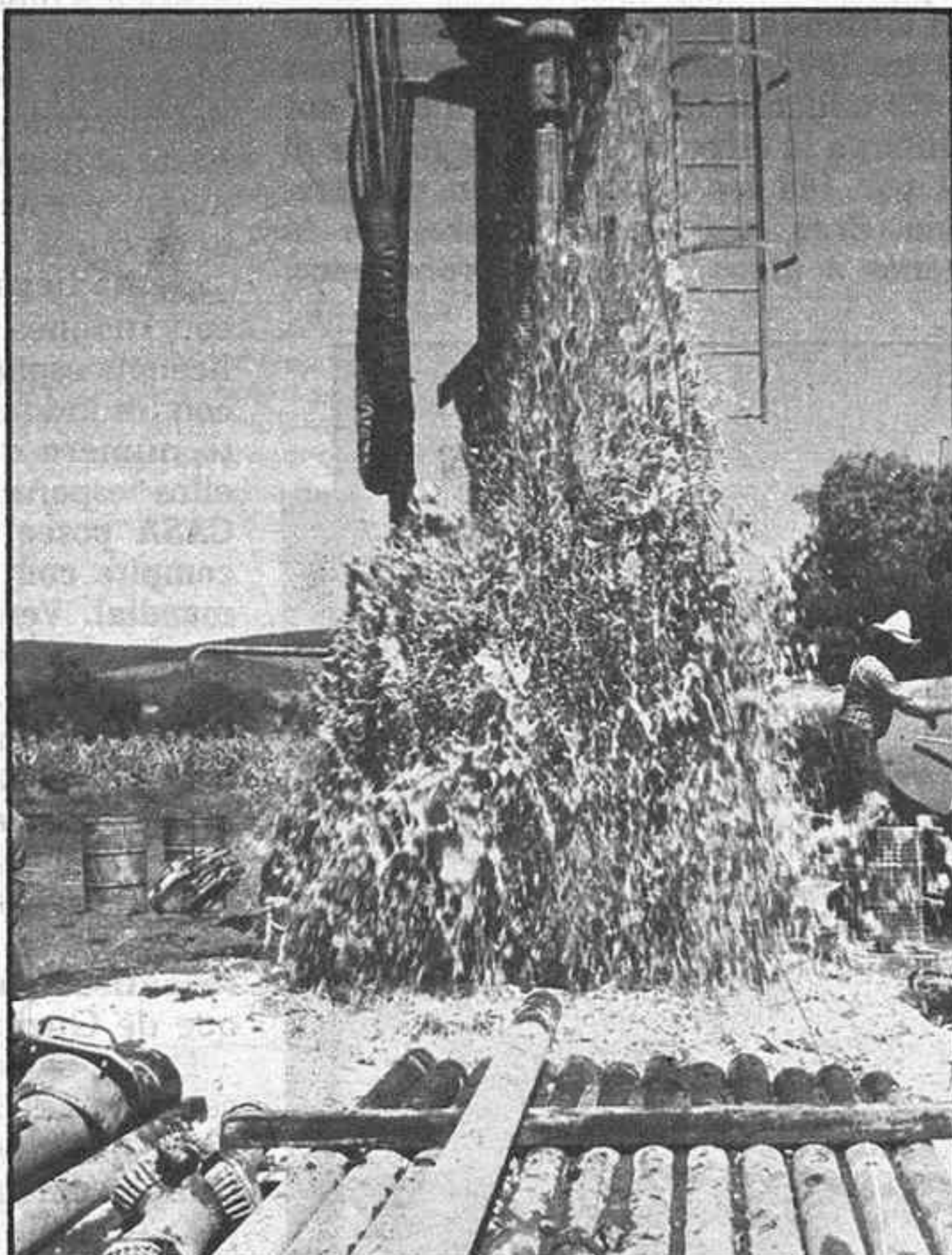
ZAHORI 1.206 trabajando en Querétaro (México) con un diámetro de 17" en terreno volcánico con intercalaciones de cenizas no consolidadas. Profundidad: 200 metros. Caudal obtenido: 60 litros por segundo
