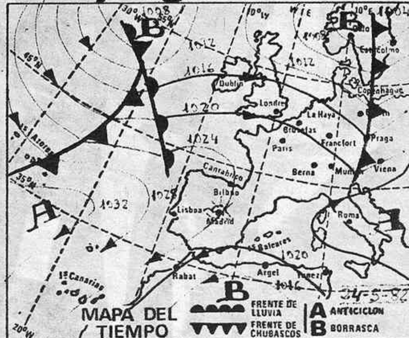
Dominio en las capas bajas de la atmósfera del régimen estable y anticiclónico, con ligera inestabilidad en el tercio norte
