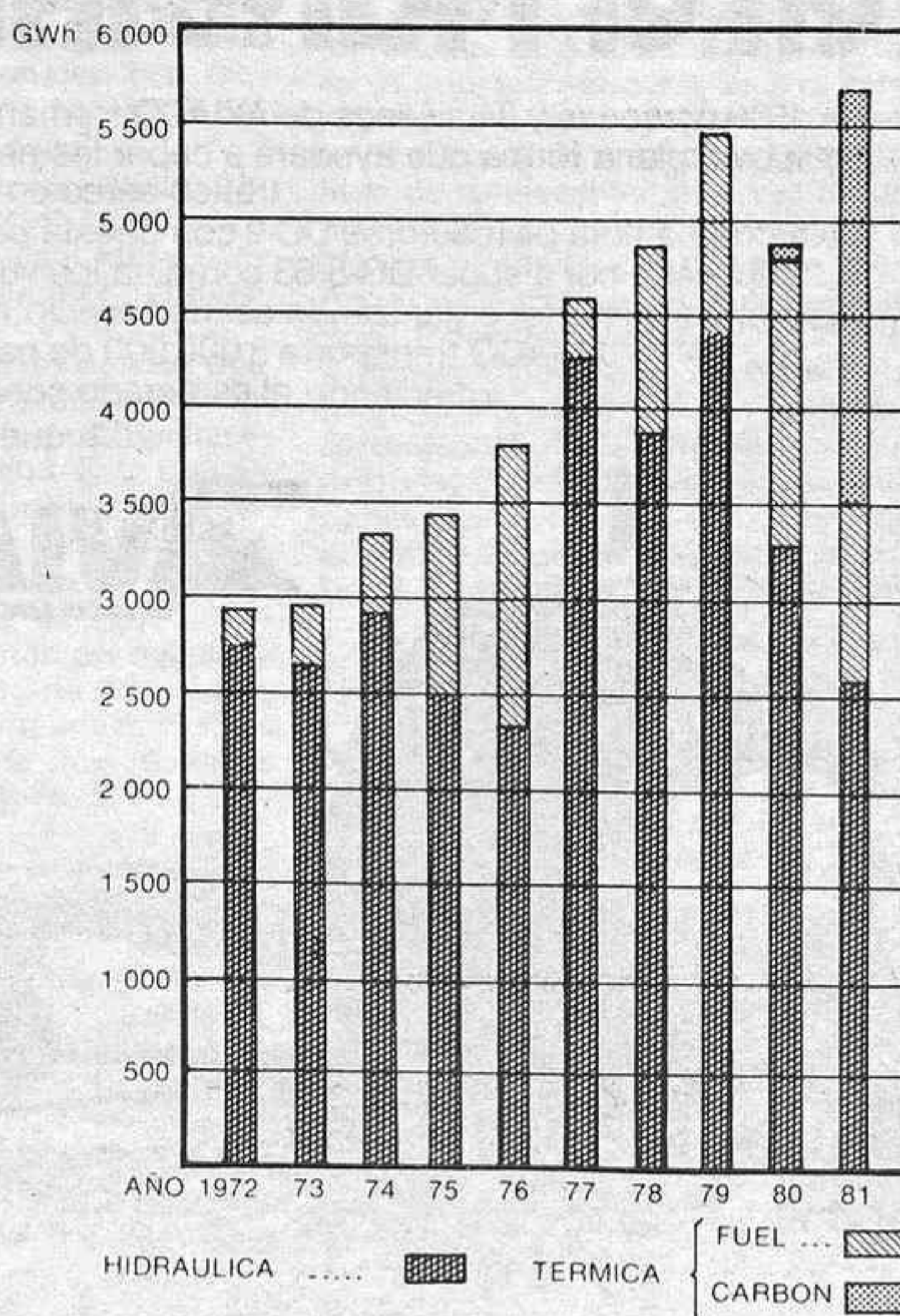
EVOLUCION DE LA PRODUCCION PROPIA HIDRAULICA Y TERMICA
