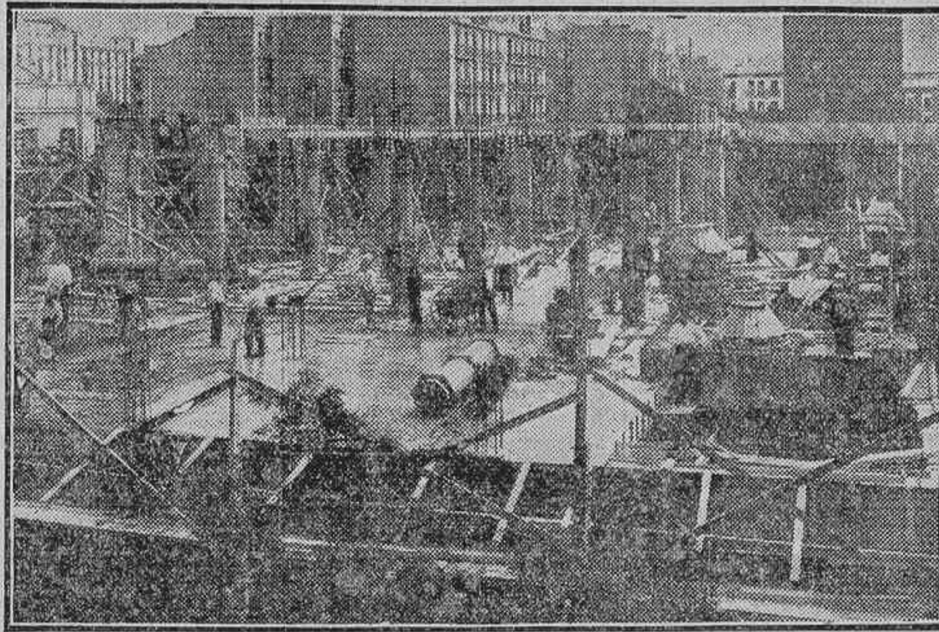
MADRID.—PREPARACION DE LOS MOLDES PARA LAS COLUMNAS DE CEMENTO EN LA SUBCENTRAL AUTOMATICA DE DELICIAS
