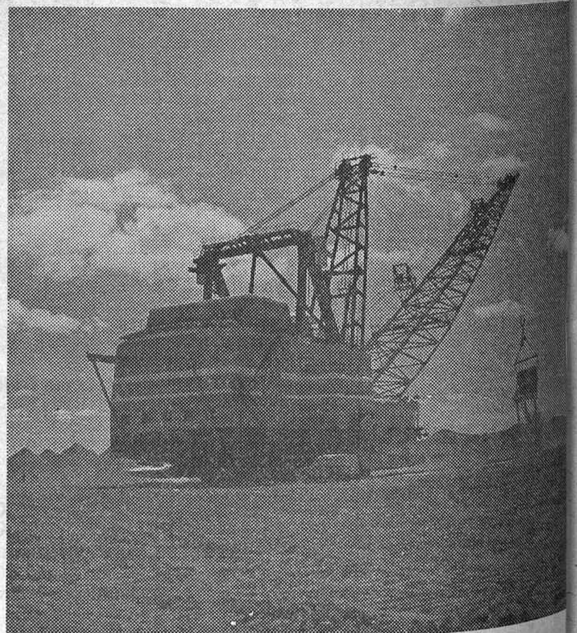
Dragolina de 46 m 3 de cangilón
