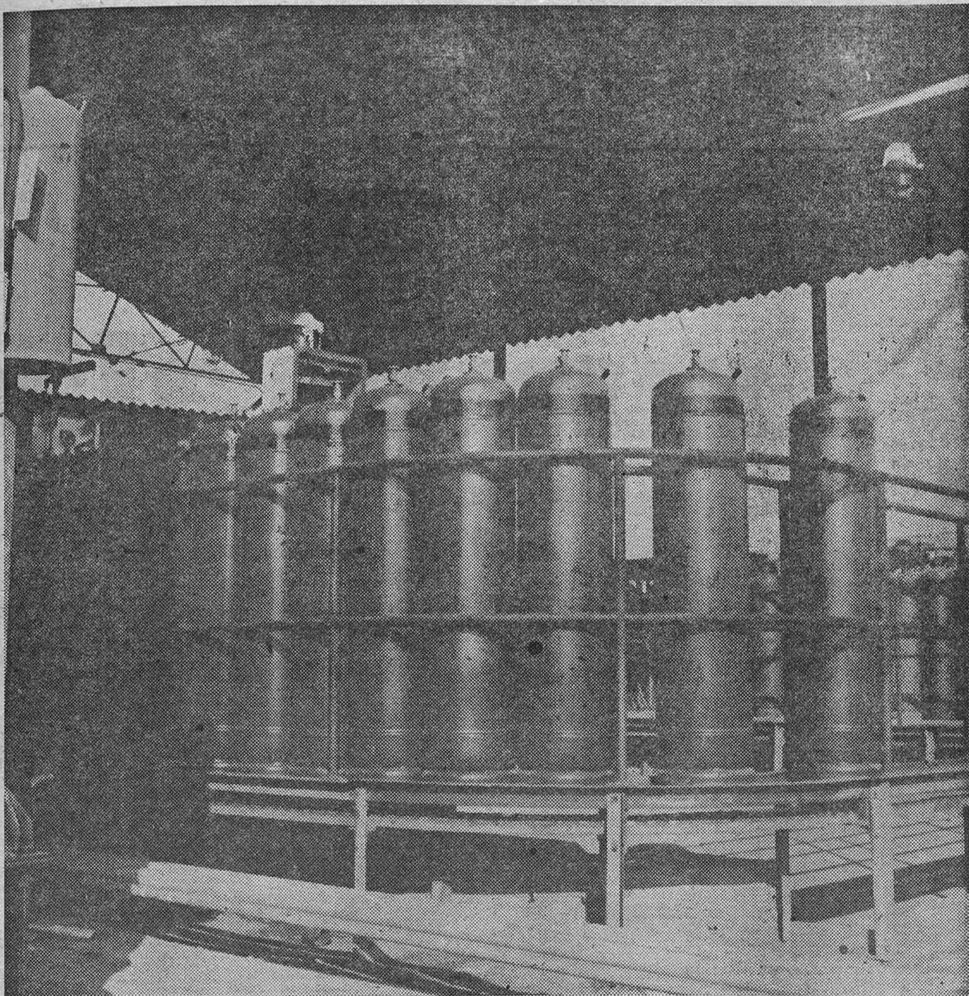
Botellas de 35 kilogramos de propano, en proceso de llenado
