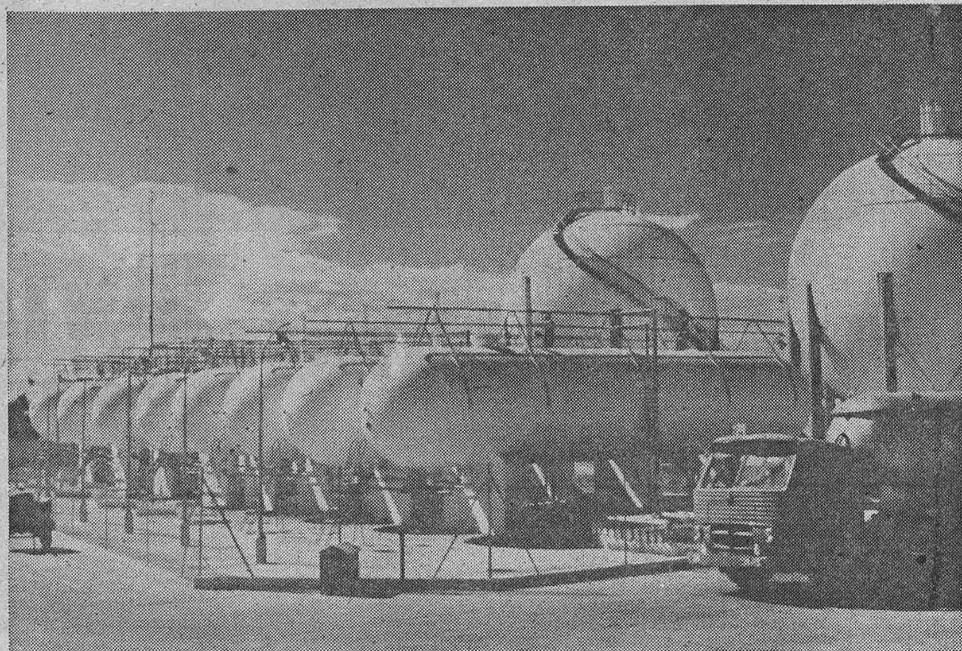
Parque de almacenaje de G. L. P. en una planta embotelladora de Butano, S. A.
