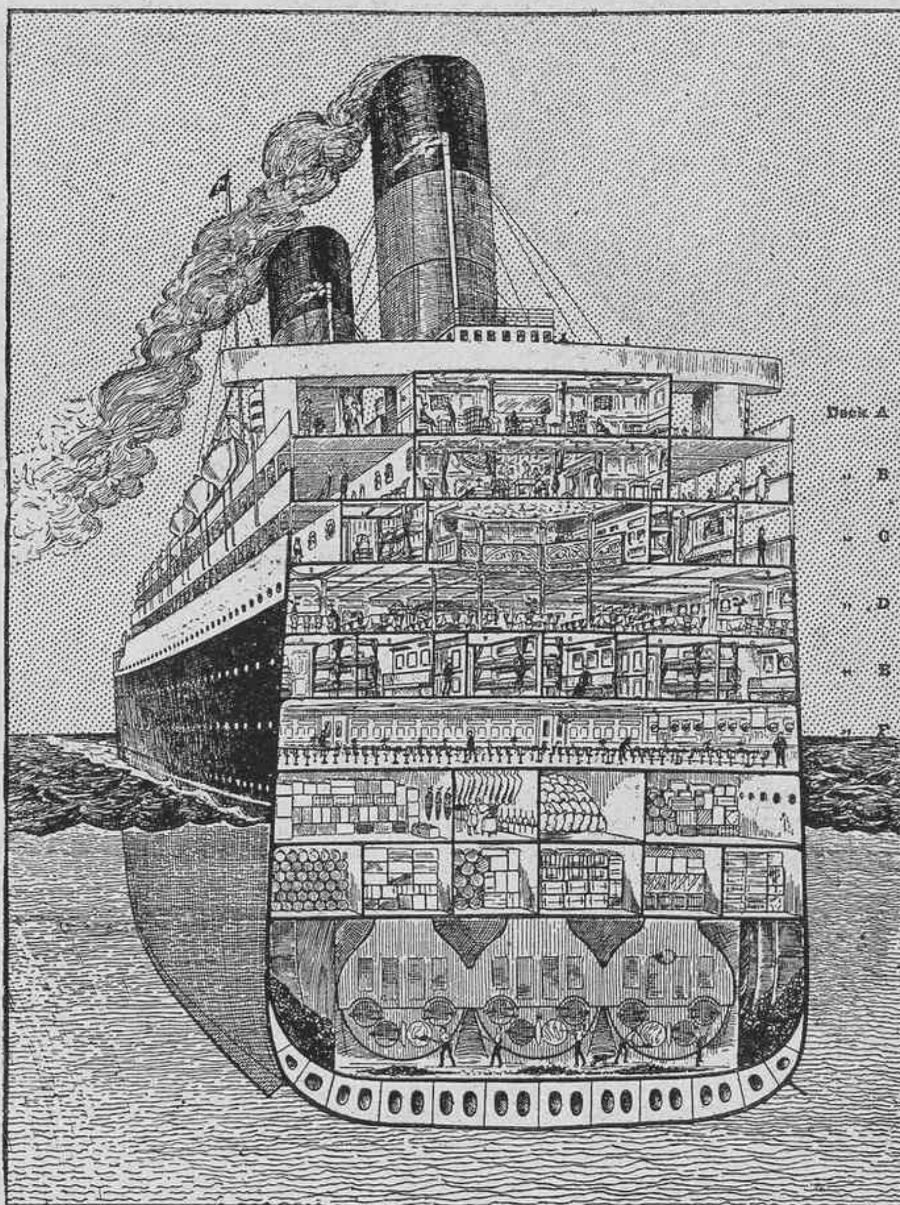
Vista de una sección del «Carmania»
