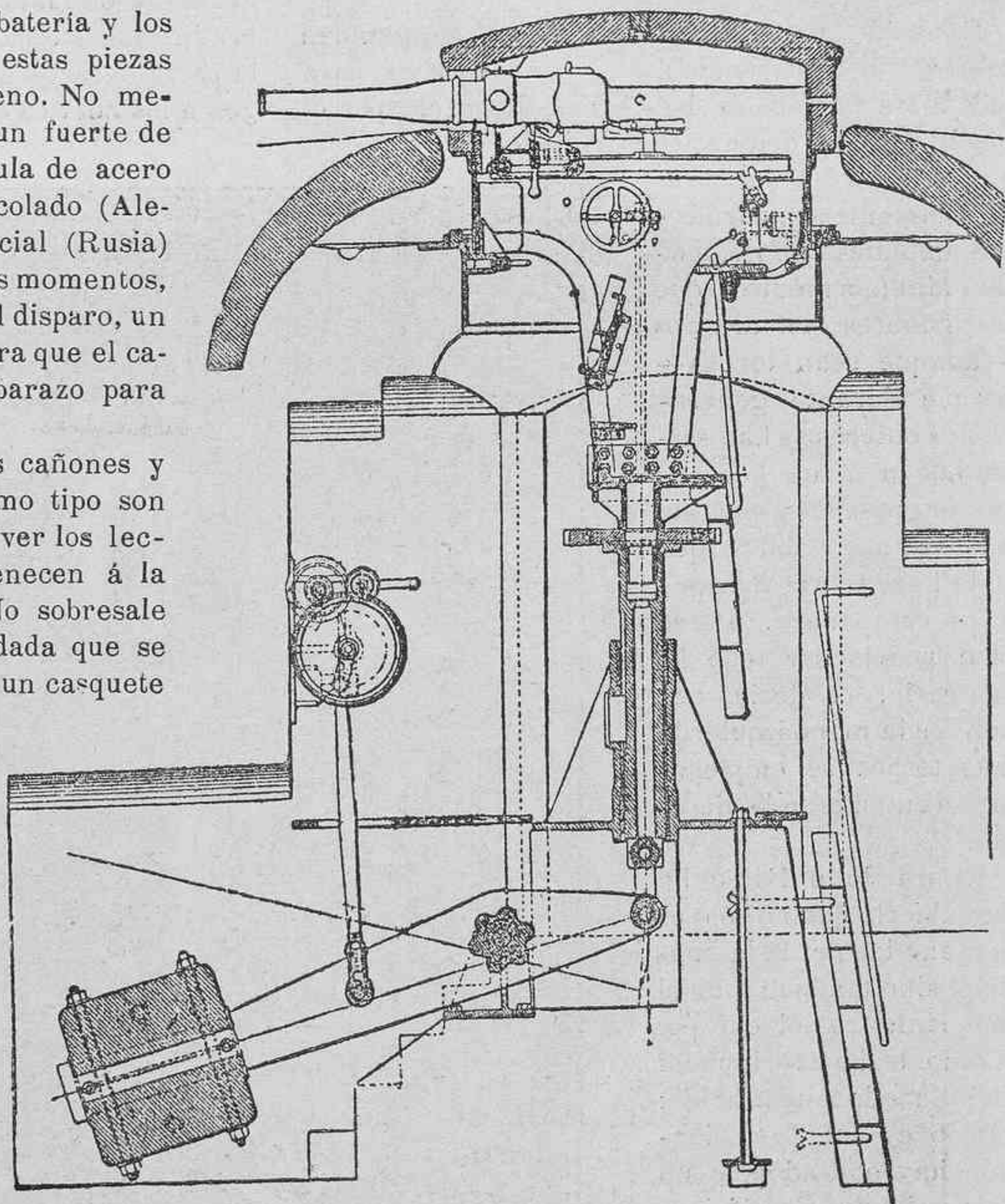
Fuerte blindado con el cañón dispuesto para disparar
