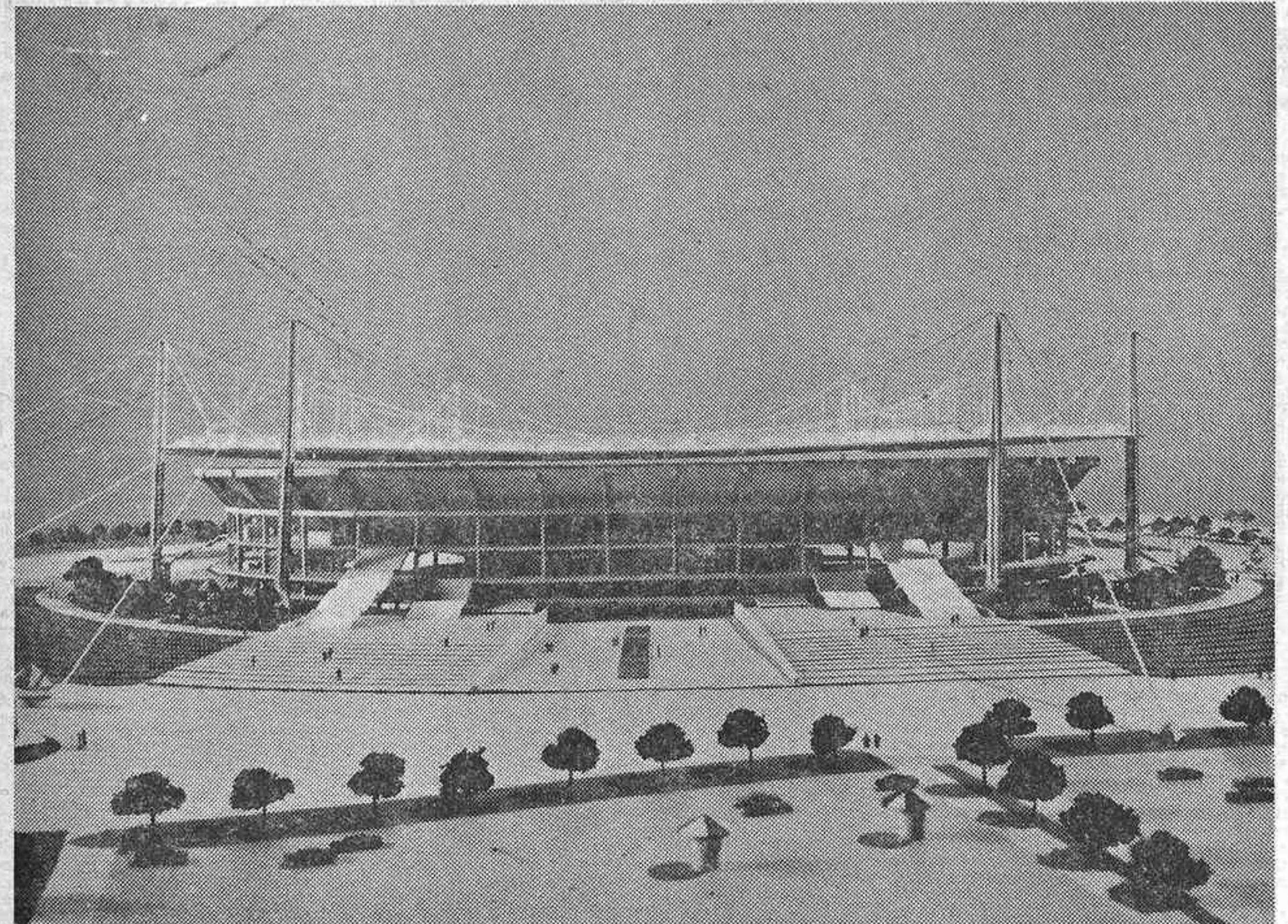
Vista lateral del anteproyecto del posible nuevo estadio del Real Madrid, obra del arquitecto Félix Candela, con capacidad para 120.000 espectadores.
