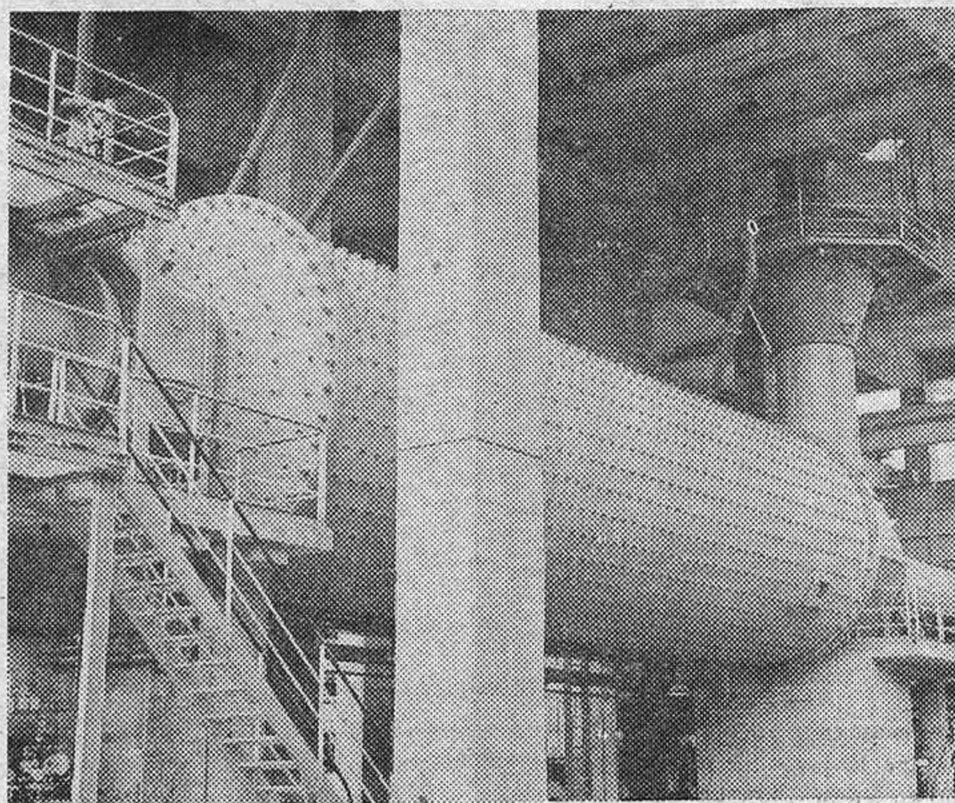
Molienda de cemento (90 t.-hora). Cementos del Cantábrico
