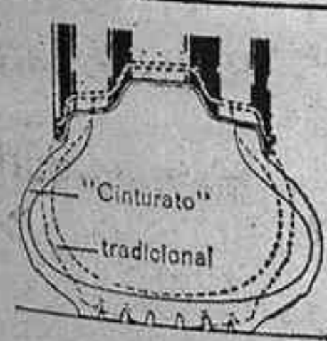
El gráfico refleja el diferente comportamiento del Cinturato comparándolo, con un neumático tradicional.
