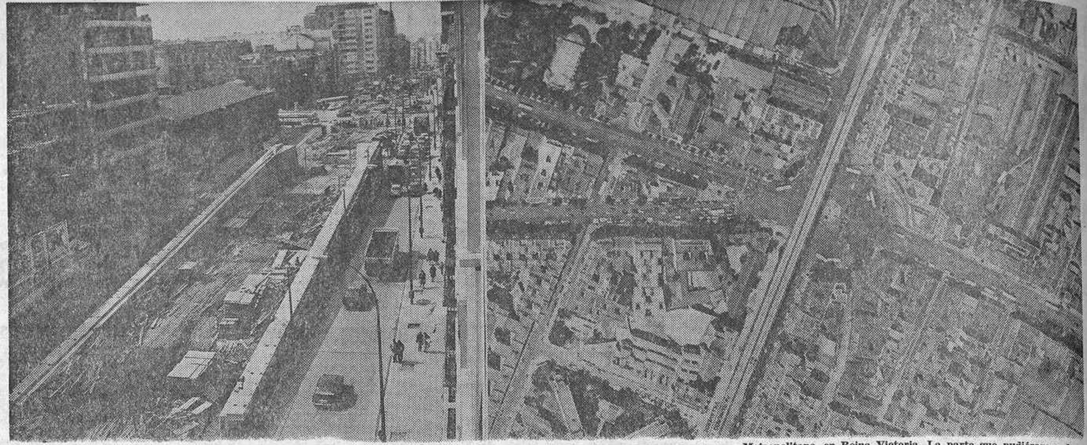
El paso elevado de Cuatro Caminos tendrá una longitud de 380 metros, desde el hospital de Maudes, en Fernández Villaverde, al cine Metropolitano, en Reina Victoria. La parte que pudéramos denominar como aérea medirá 154 metros y estará sustentada en 34 pilotes. En los grabados puede verse el estado de las obras y el puen te simulado sobre la glorieta de Cuatro Caminos. (Foto L. Jiménez.)
