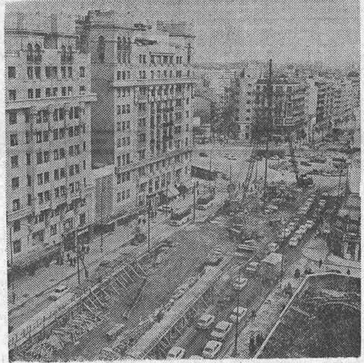
El tipo de máquina para la realización del pilotaje es el más moderno que existe. Es como una torre colosal, que cuando entra en actividad se convierte en un espectáculo para los viandantes de Cuatro Caminos. (Foto L. Jiménez.)
