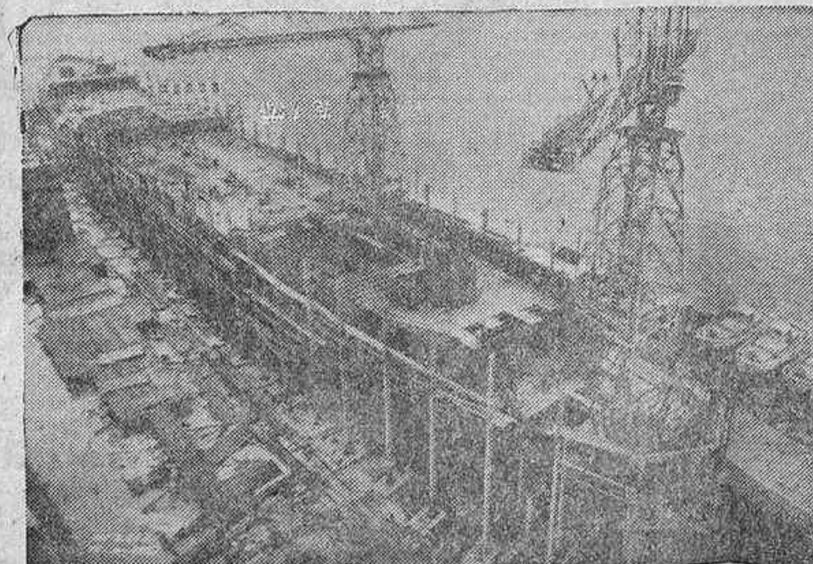
EL FERROL DEL CAUDILLO.—Petrolero «Almirante F. Moreno» de 14.000 Tm., en gradas, construido por la Empresa Nacional «Bazán»
