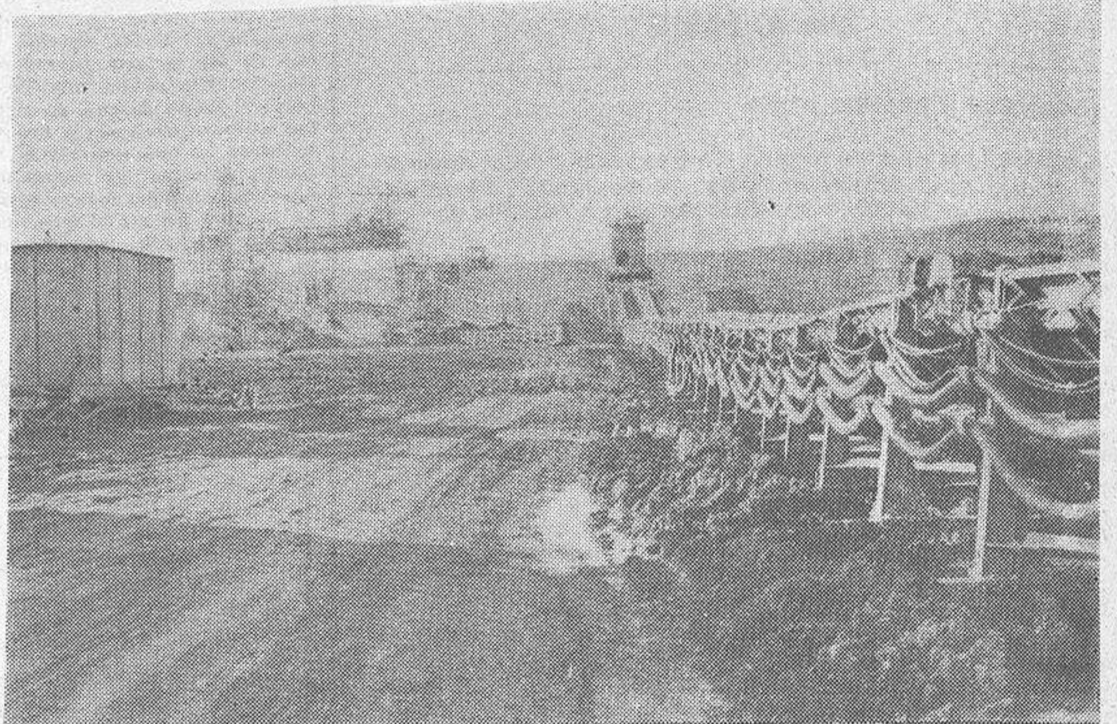
He aquí una de las explotaciones gallegas de lignitos. A ella, así como a otra de las existentes, vendrá a unirse la bolsa que acaba de descubrirse en la antigua laguna de Antela.
