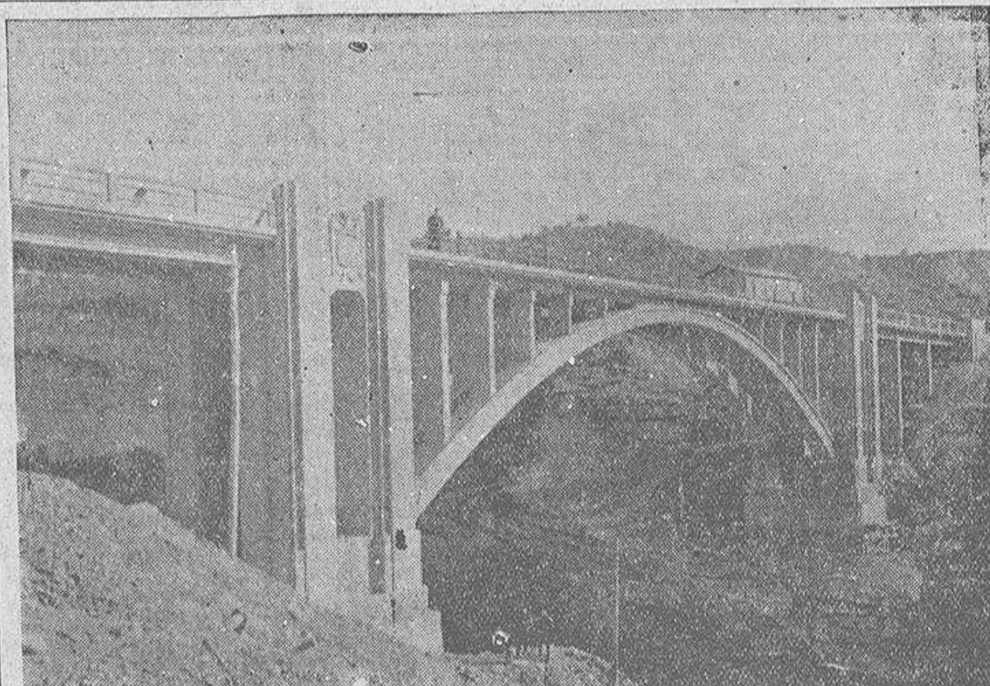
Un alarde de la ingeniería española. Puente Arbox. — El teniente coronel de Ingenieros, señor Arbox que murió en actos del servicio el 1 de diciembre de 1938, fue autor de esta maravilla de la ingeniería española que se construyó tan solo en 96 días de trabajo. Como homenaje a la memoria del ilustre ingeniero, nos honramos con este trabajo
