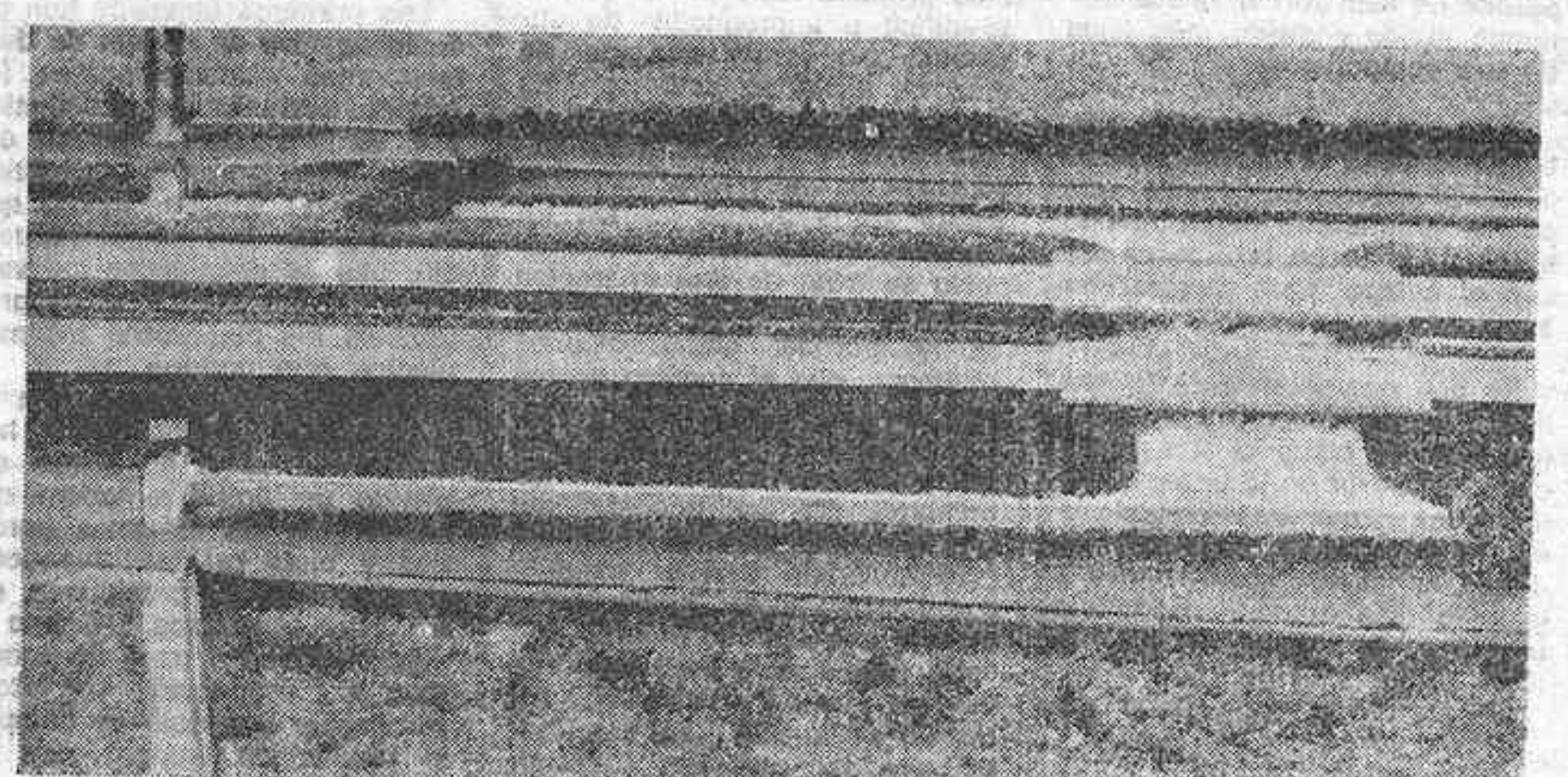
Maqueta del cruce de la autopista con el Burseral. En la parte inferior se aprecia el proyecto de muro de defensa.
