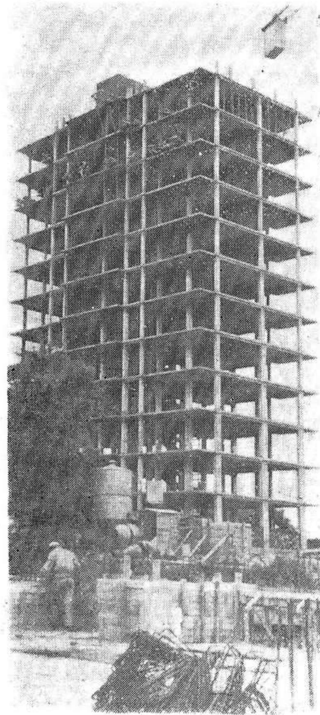
Planta baja y once alturas de hormigón armado que ya se levantan en una de las torres del Conjunto Residencial «El Mirador del Doncel». En las obras reina una gran actividad, ya que en un plazo fijado de 18 a 24 meses hay que dar por terminadas totalmente las obras.
