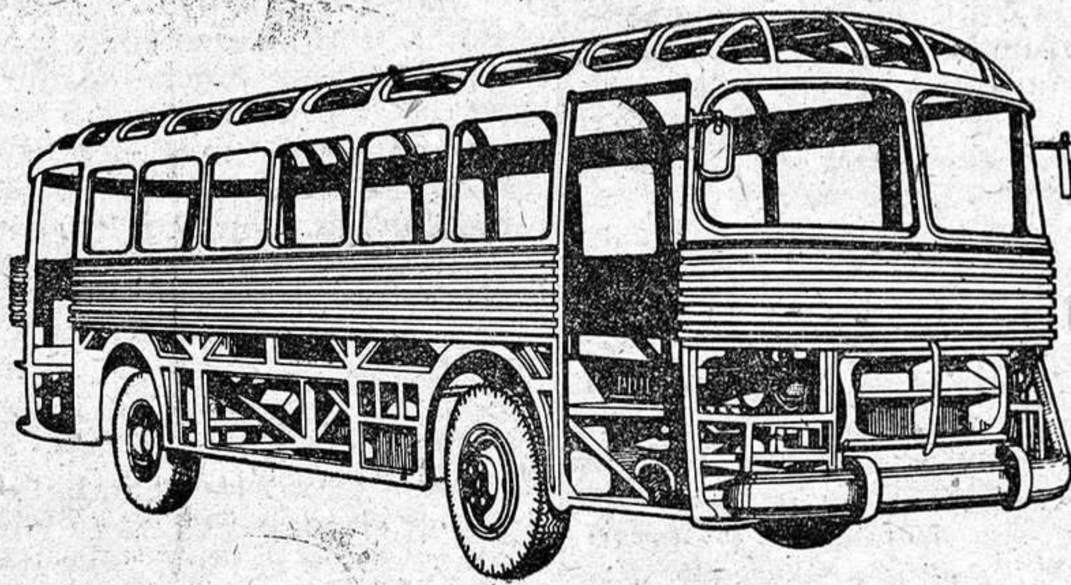
AUTOBASTIDOR: ESTRUCTURA MONOCASCO
