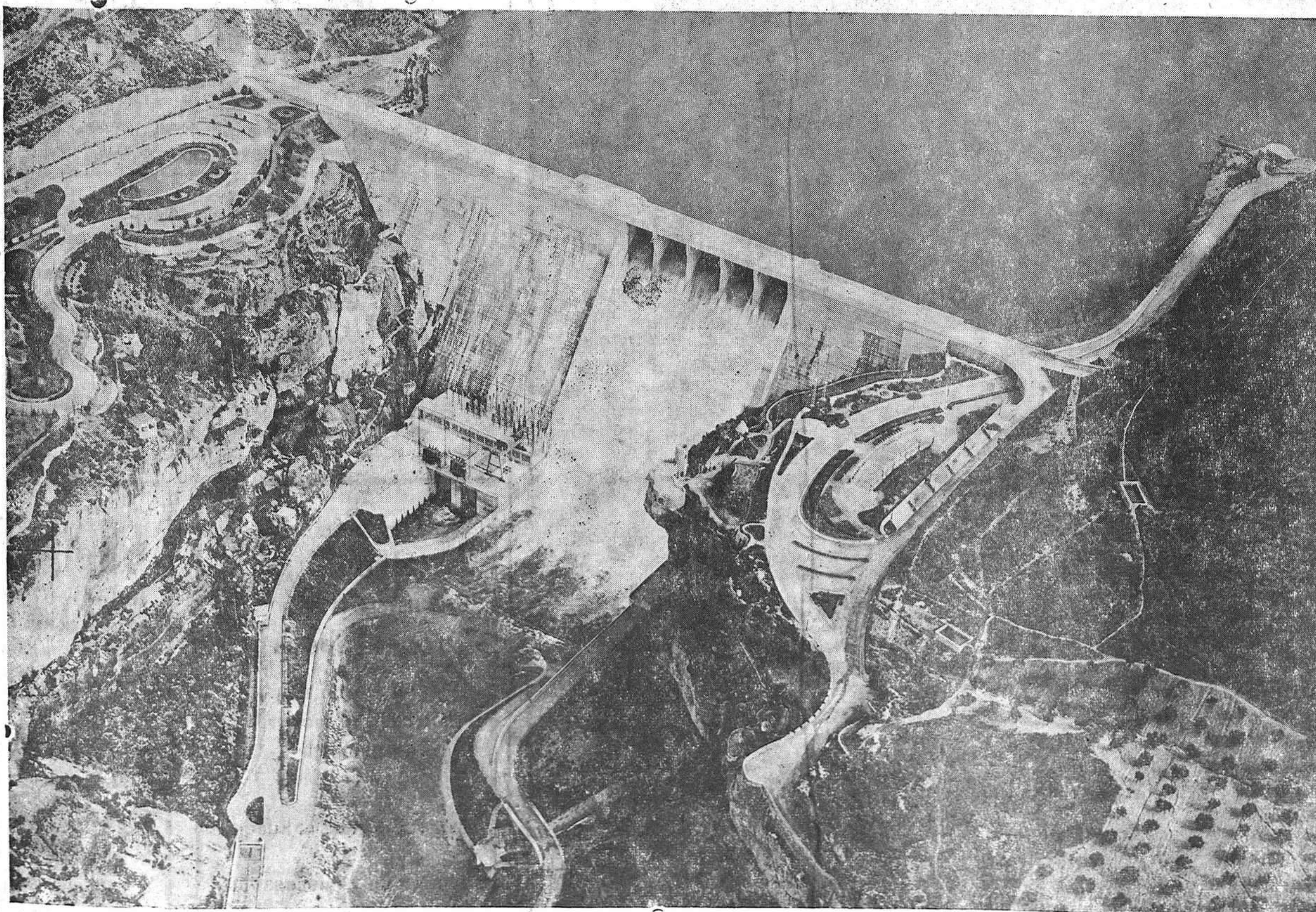
ENTREPEÑAS: VISTA AEREA DEL EMBALSE, PRESA Y CENTRAL
