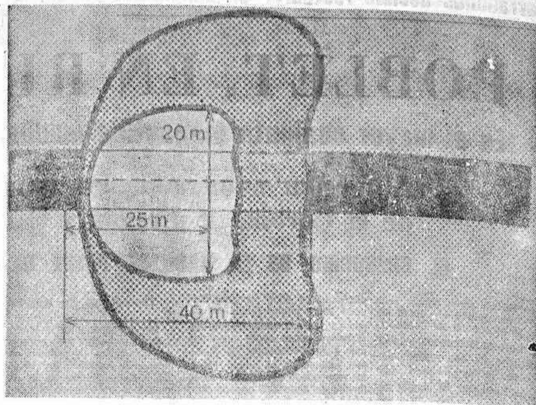
Grafico comparativo del haz de luz de un faro normal y de un proyector antiniebla CIBIE
