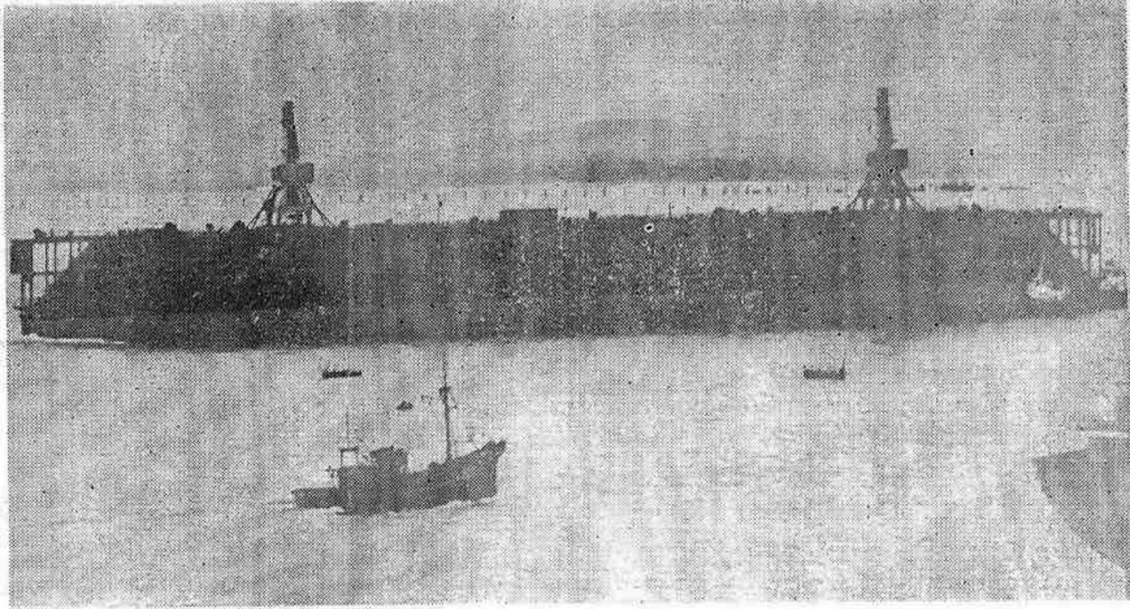
SANTANDER. — Dique flotante para Méjico, construido en la factoría de Astilleros de Santander...
