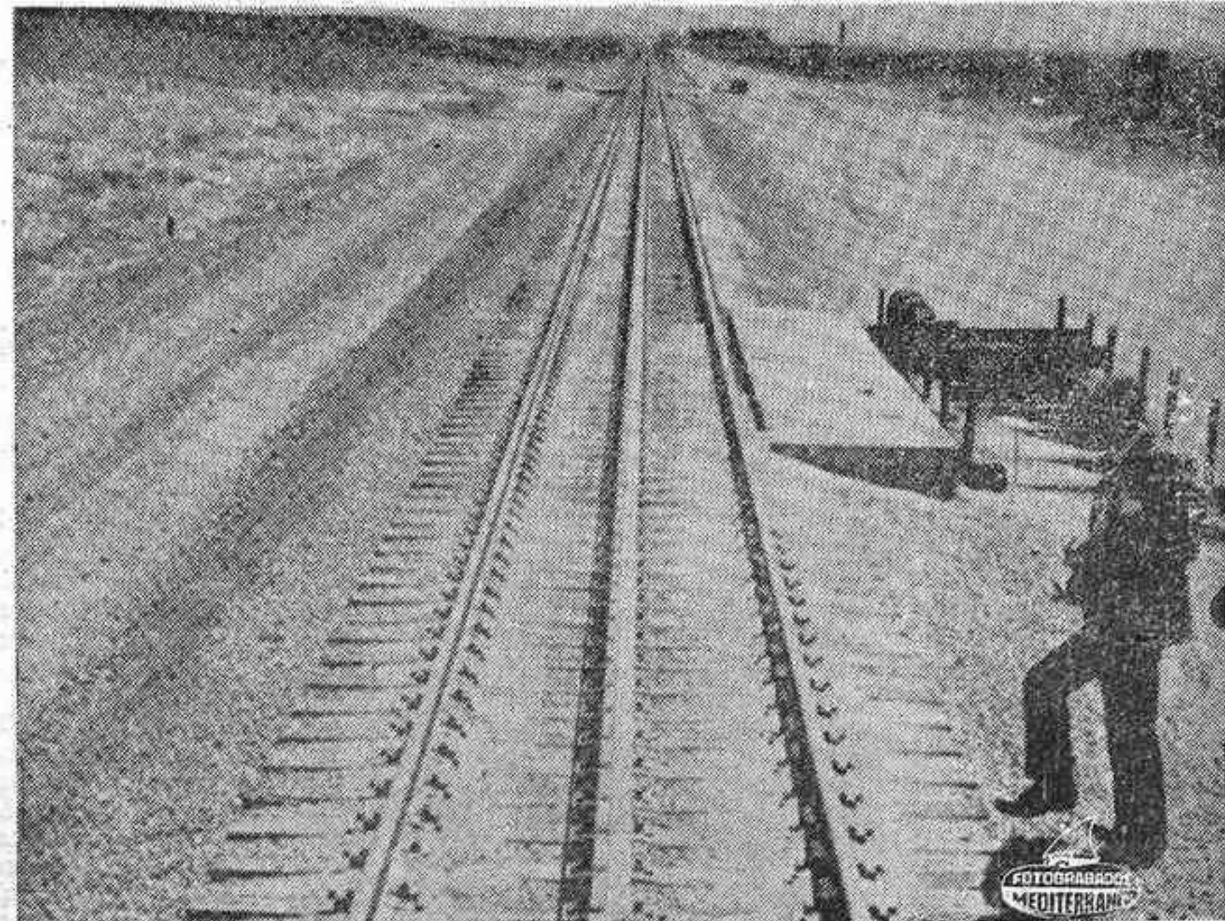
La vía del recinto de ensayo. En el centro, la placa de aluminio que asegura el funcionamiento del motor lineal.— (Foto PYRESA)
