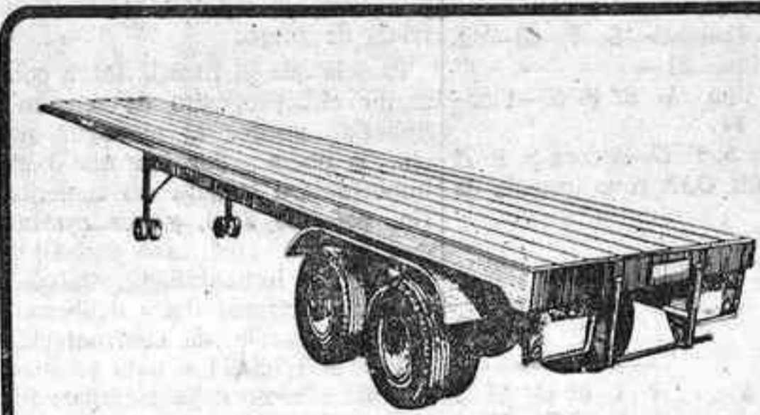
Carga útil 27 Tm.
