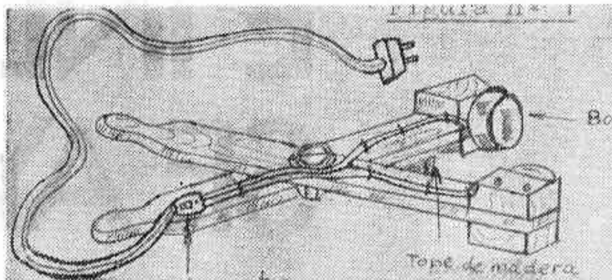
1. Diseño de la tenaza
