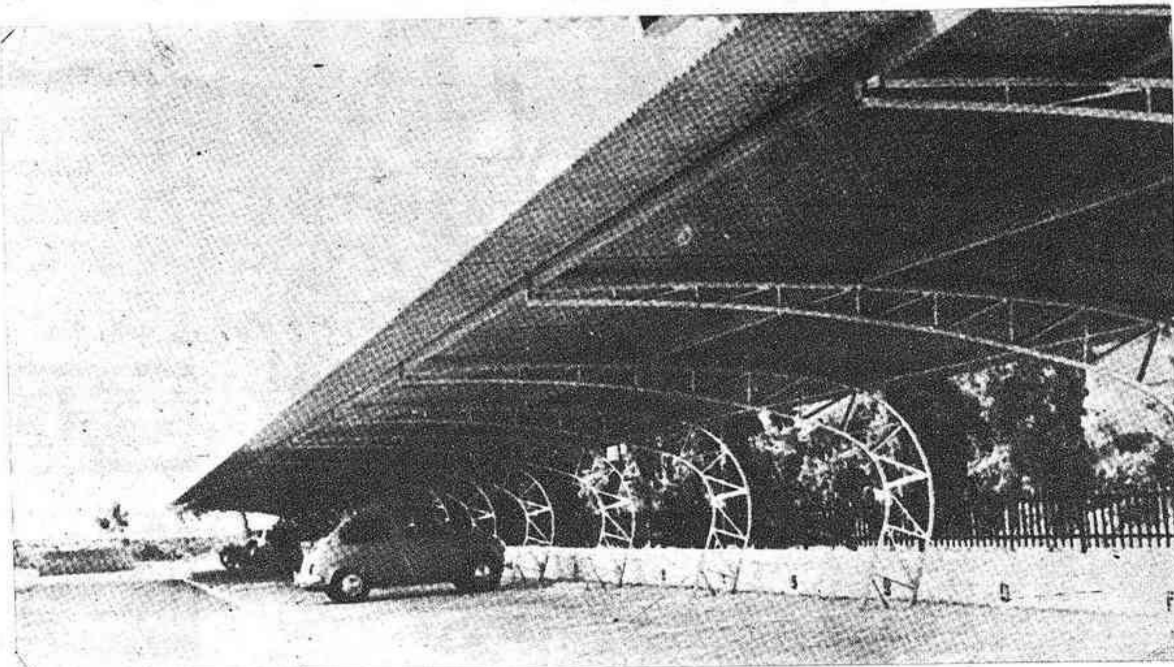
Aparcamientos metálicos para vehículos
