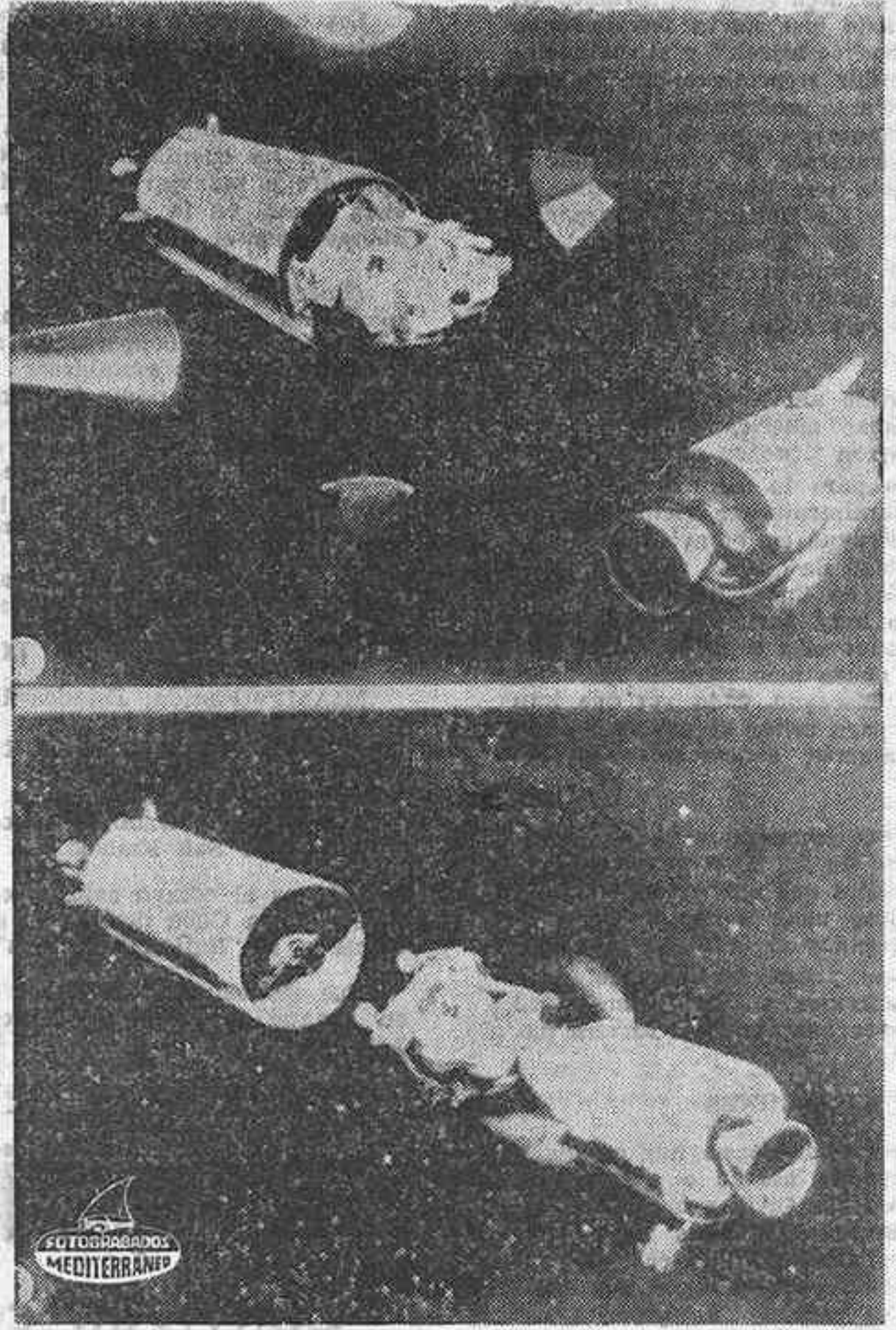
WASHINGTON. — Dibujos en los que se muestran el módulo lunar que se posará en la Luna con motivo de la misión «Apolo XI» en la que se pretende que dos astronautas pongan pie en dicho satélite mientras un tercer astronauta permanecerá en el módulo comando en espera de su regreso. — (Telefoto UPI-CIFRA)
