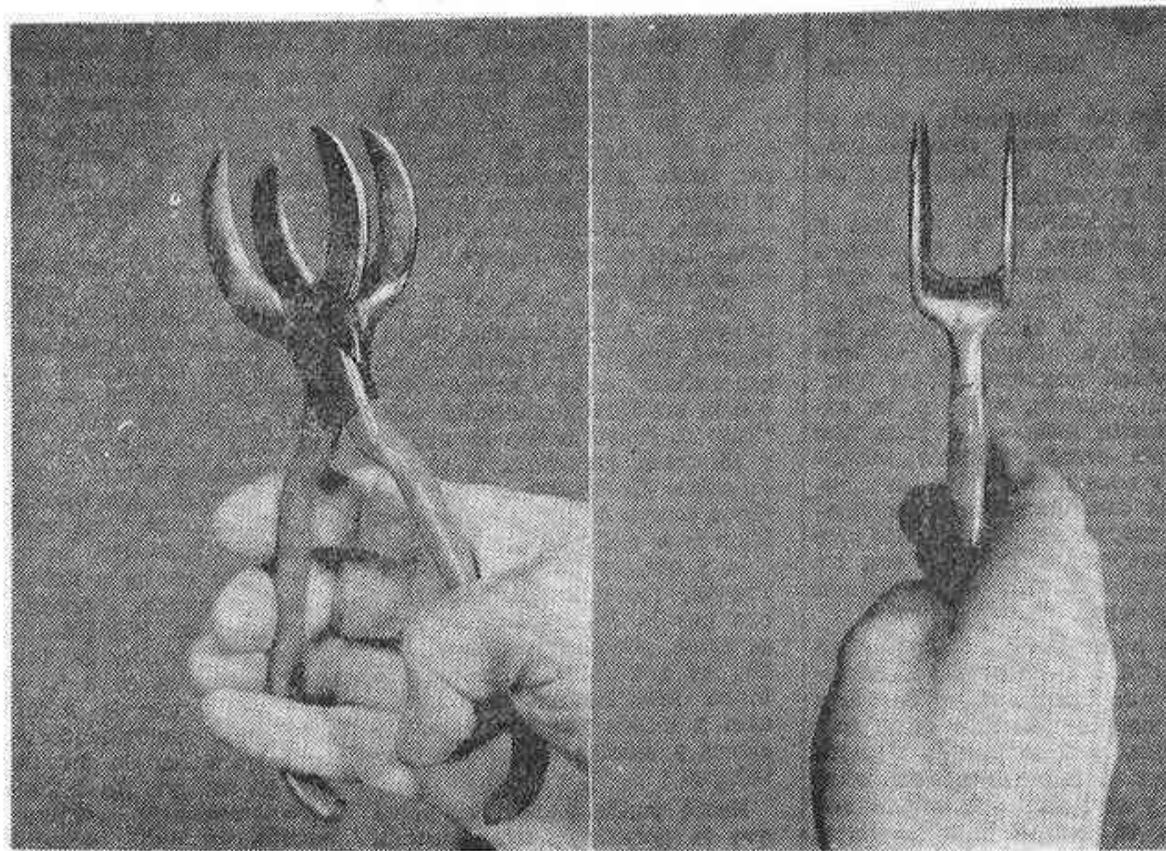
Tijera de doble corte para facilitar la realización del anillo invertido
