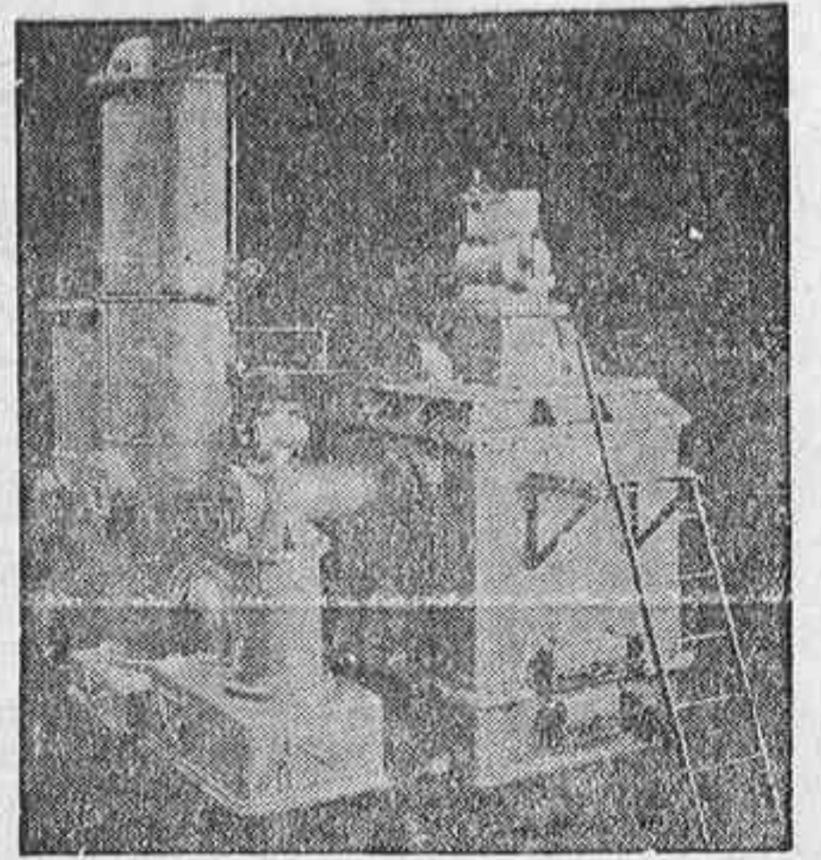
Gasógeno sencillo
