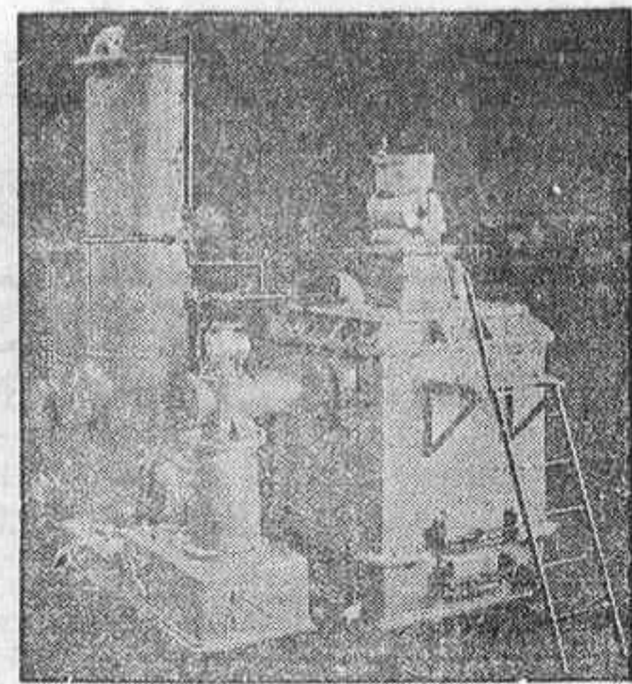
Gasógeno sencillo
