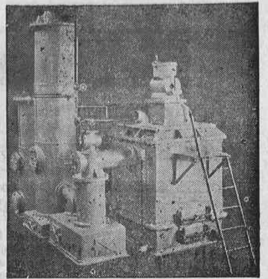
Gasógeno sencillo
