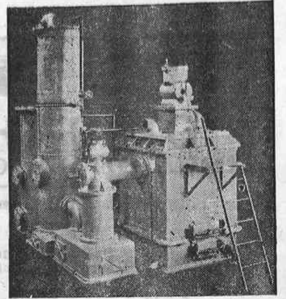
Gasógeno sencillo
