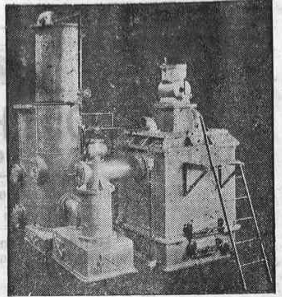
Gasógeno sencillo
