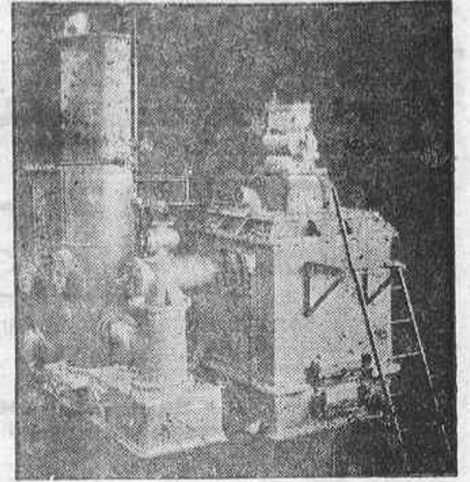
Gasógeno sencillo
