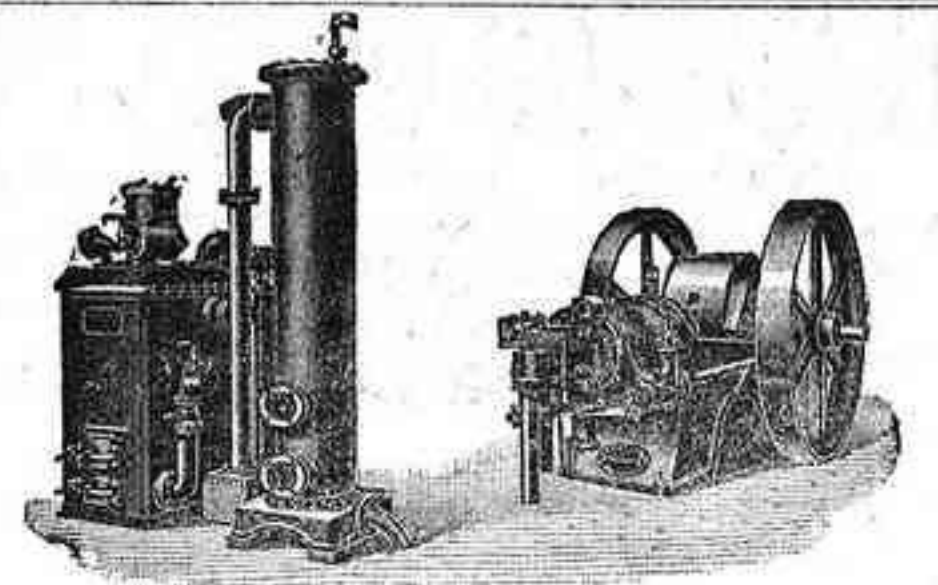
Motor y Gasógeno (Gas pobre)
