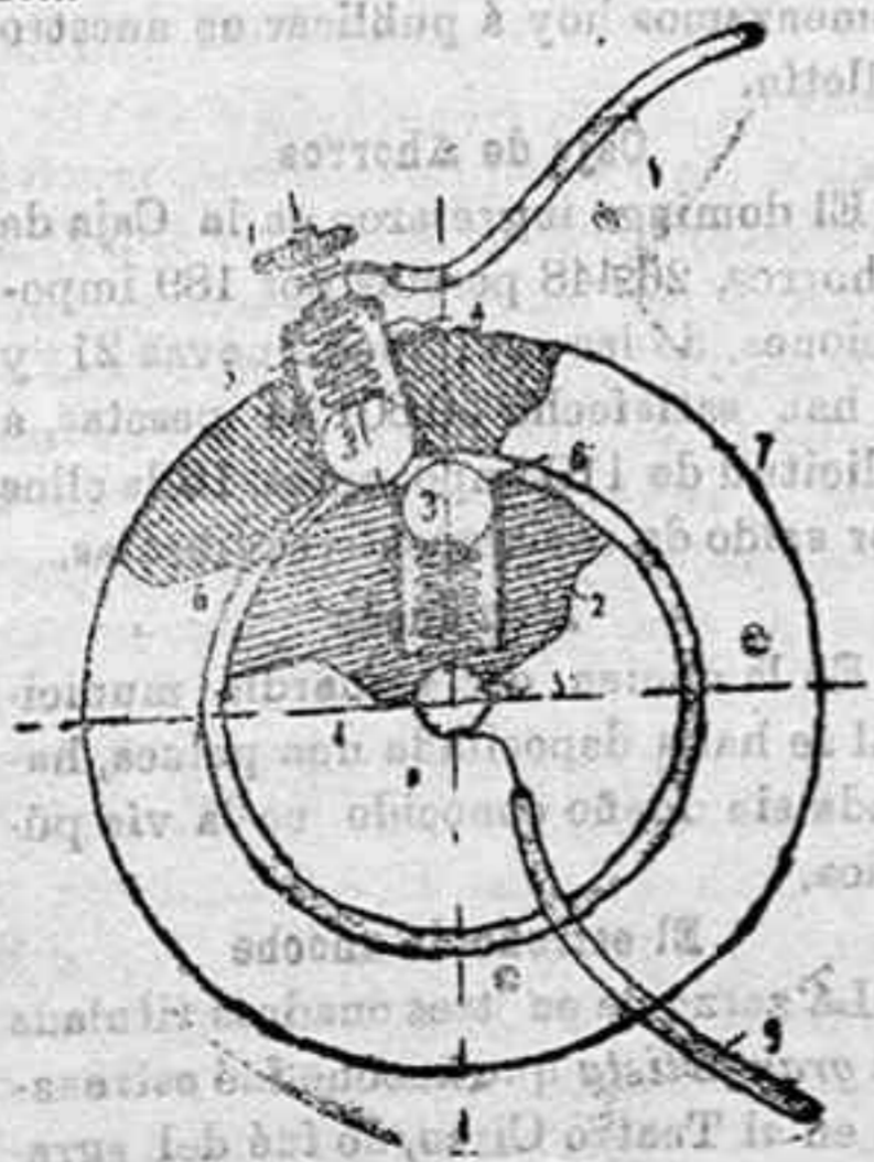
Interruptor eléctrico
