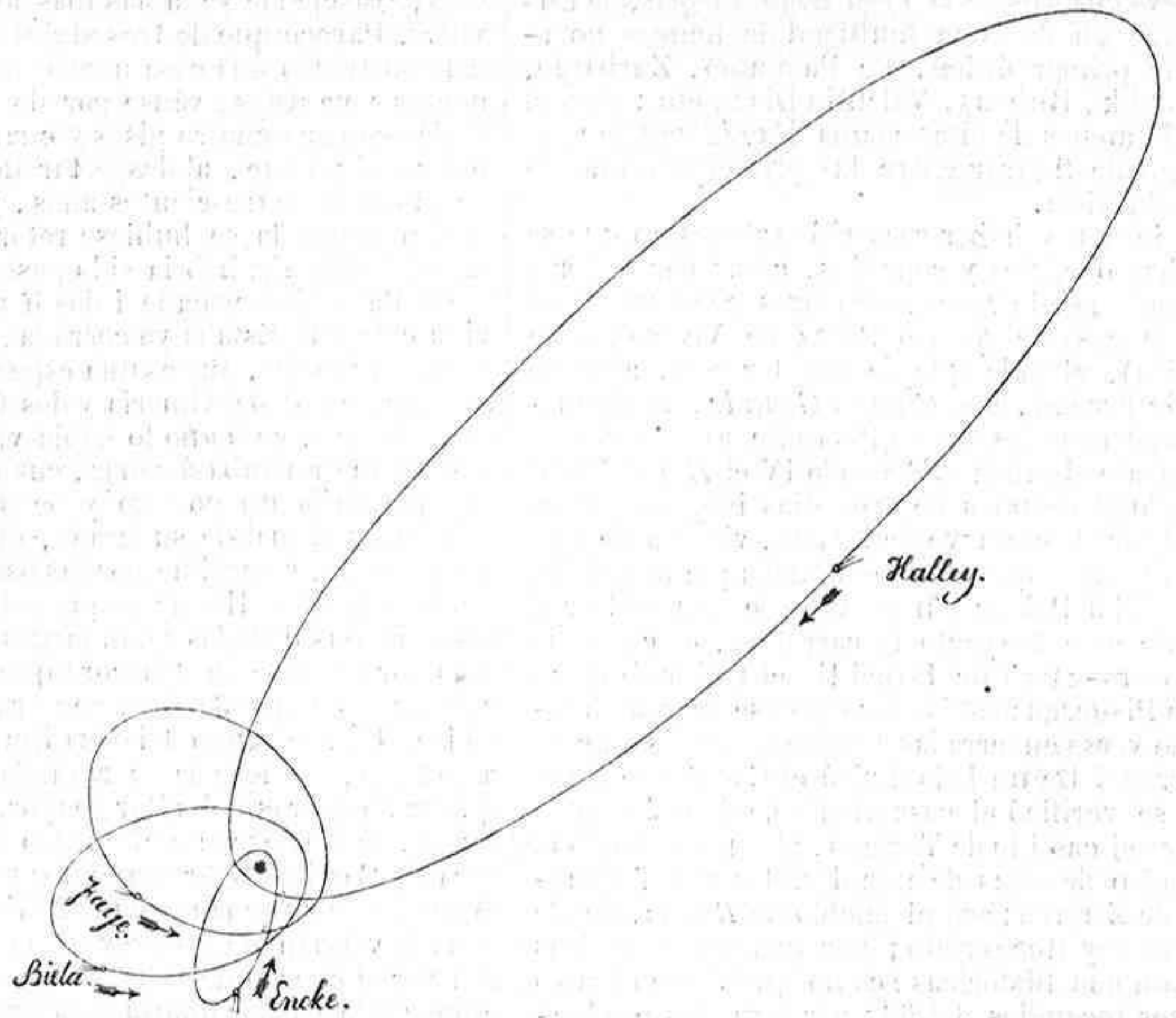
Fig. 7.—Orbitas de los cometas de Halley, Encke, Biela y Faye.
