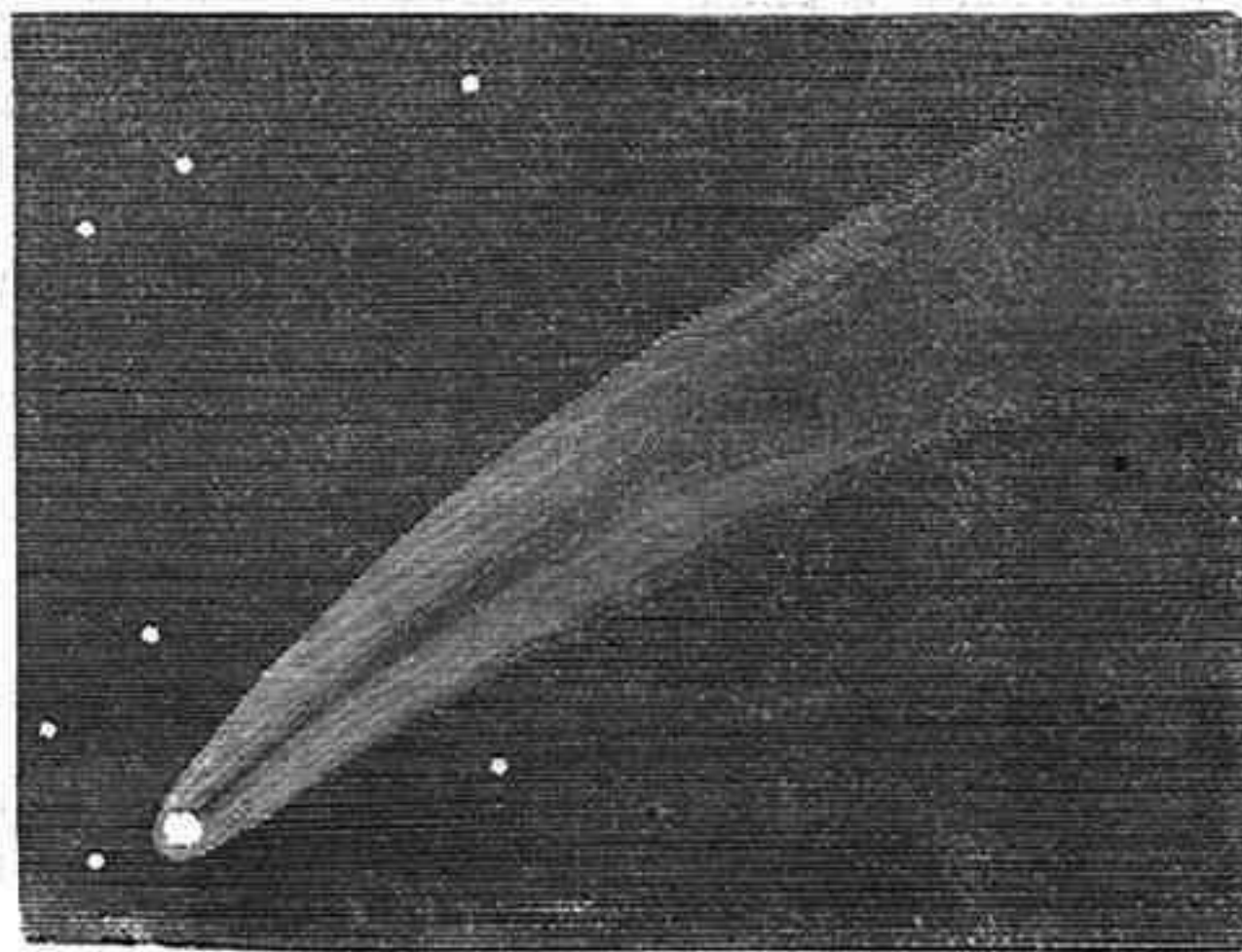
Fig. 9.—Cometa de Donati.
