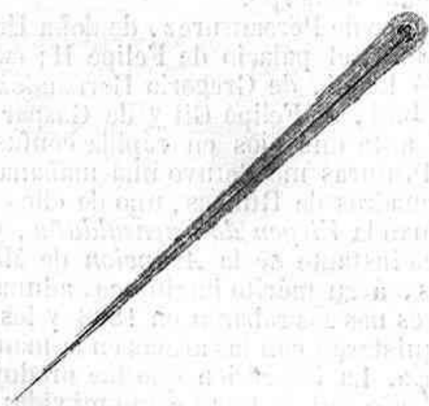
Fig. 1.—Cometa de Halley.
