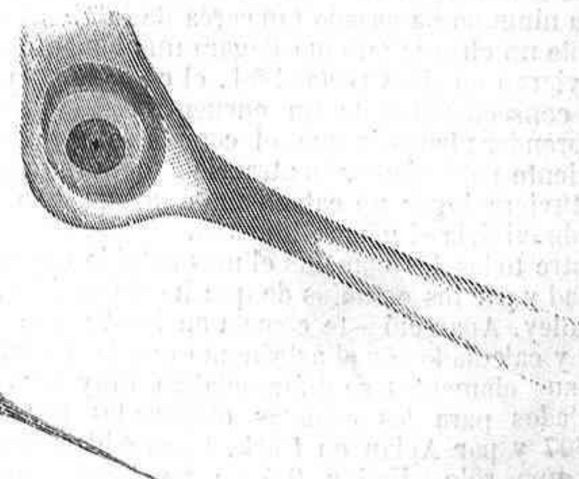
Fig. 5.—Cometa de Biela
