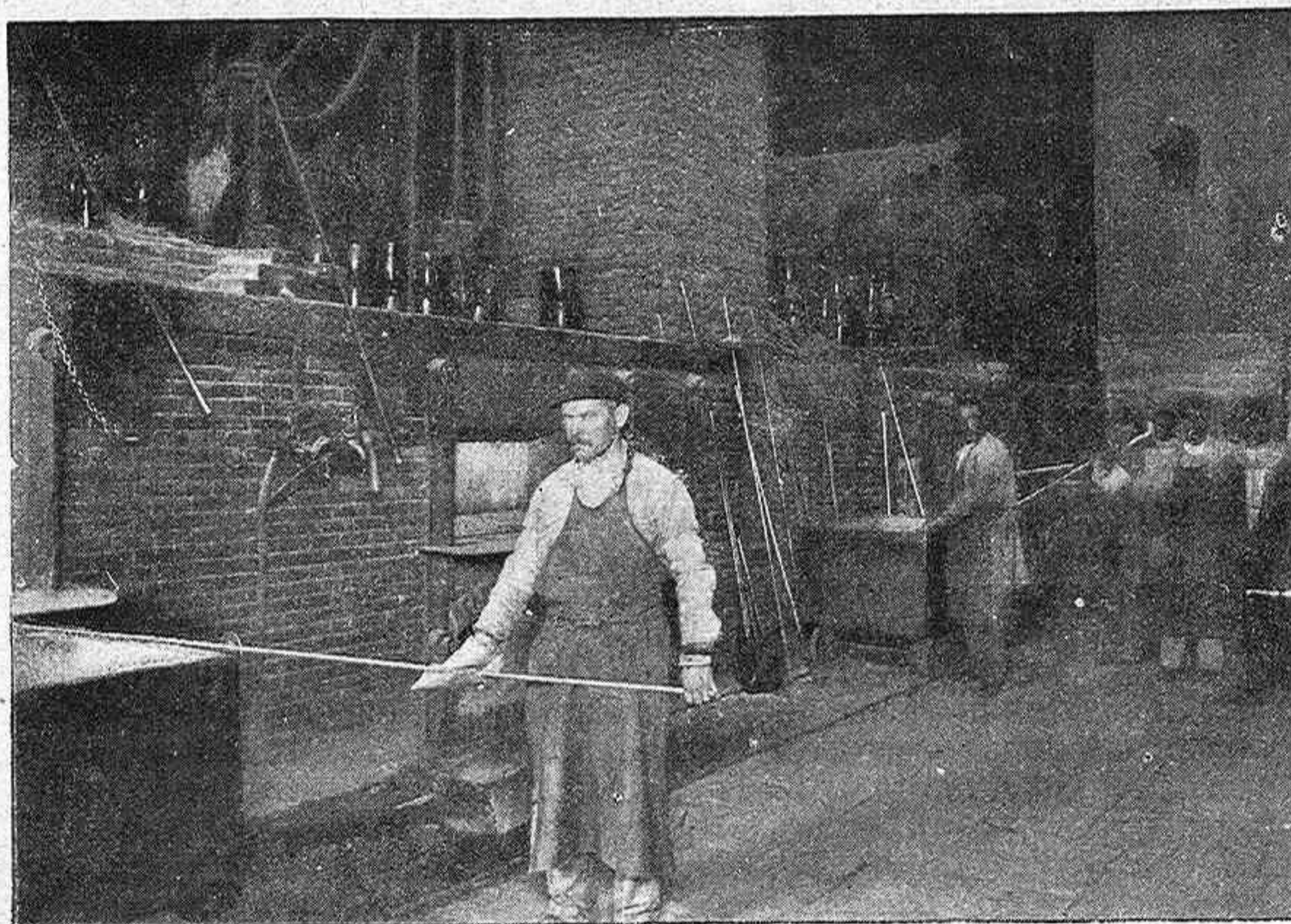
HORNOS DE RECOCHO
