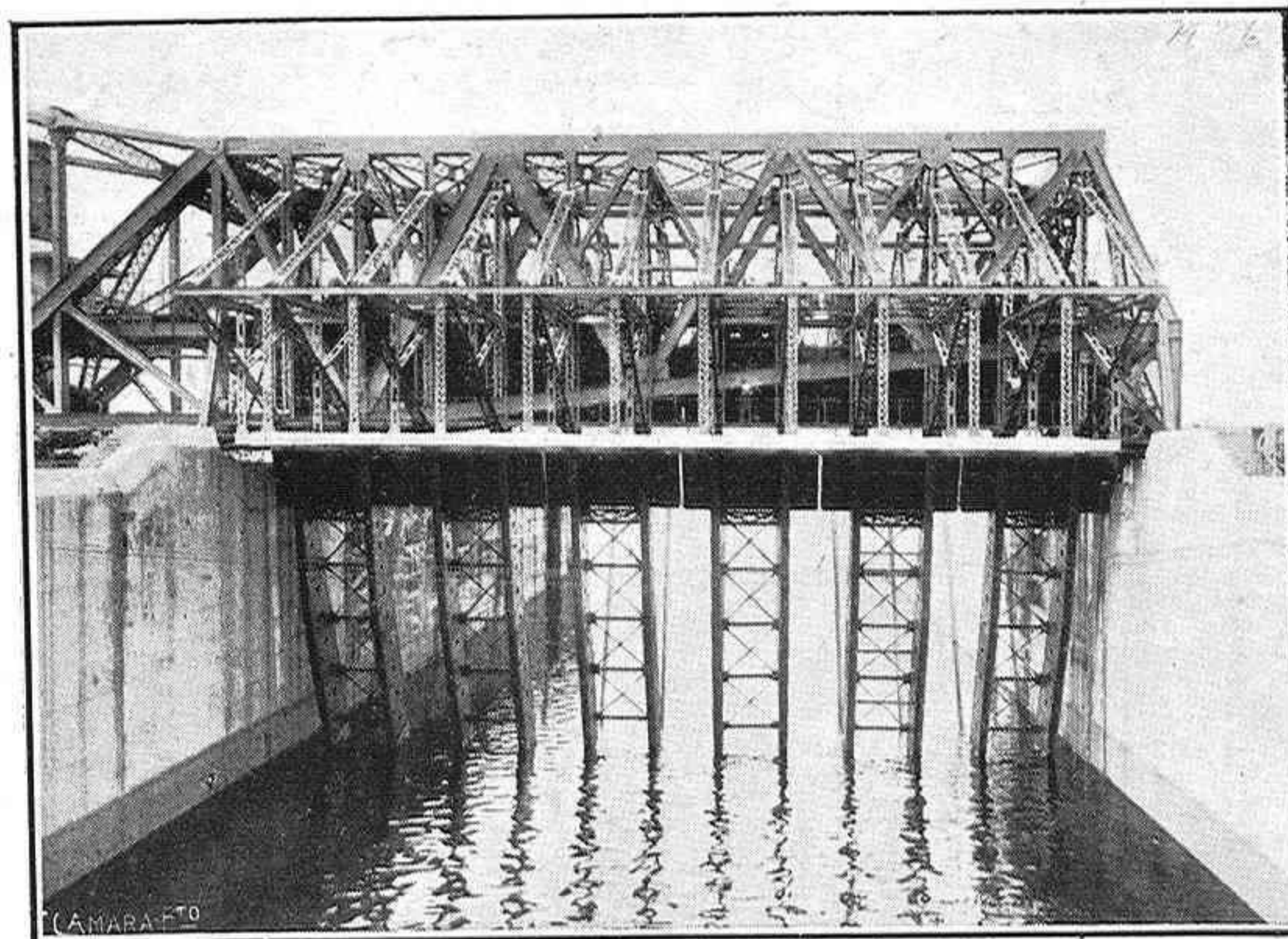
Dique de emergencia en la primera posición de servicio, por si se rompieran los dos juegos de compuertas de cada esclusa
