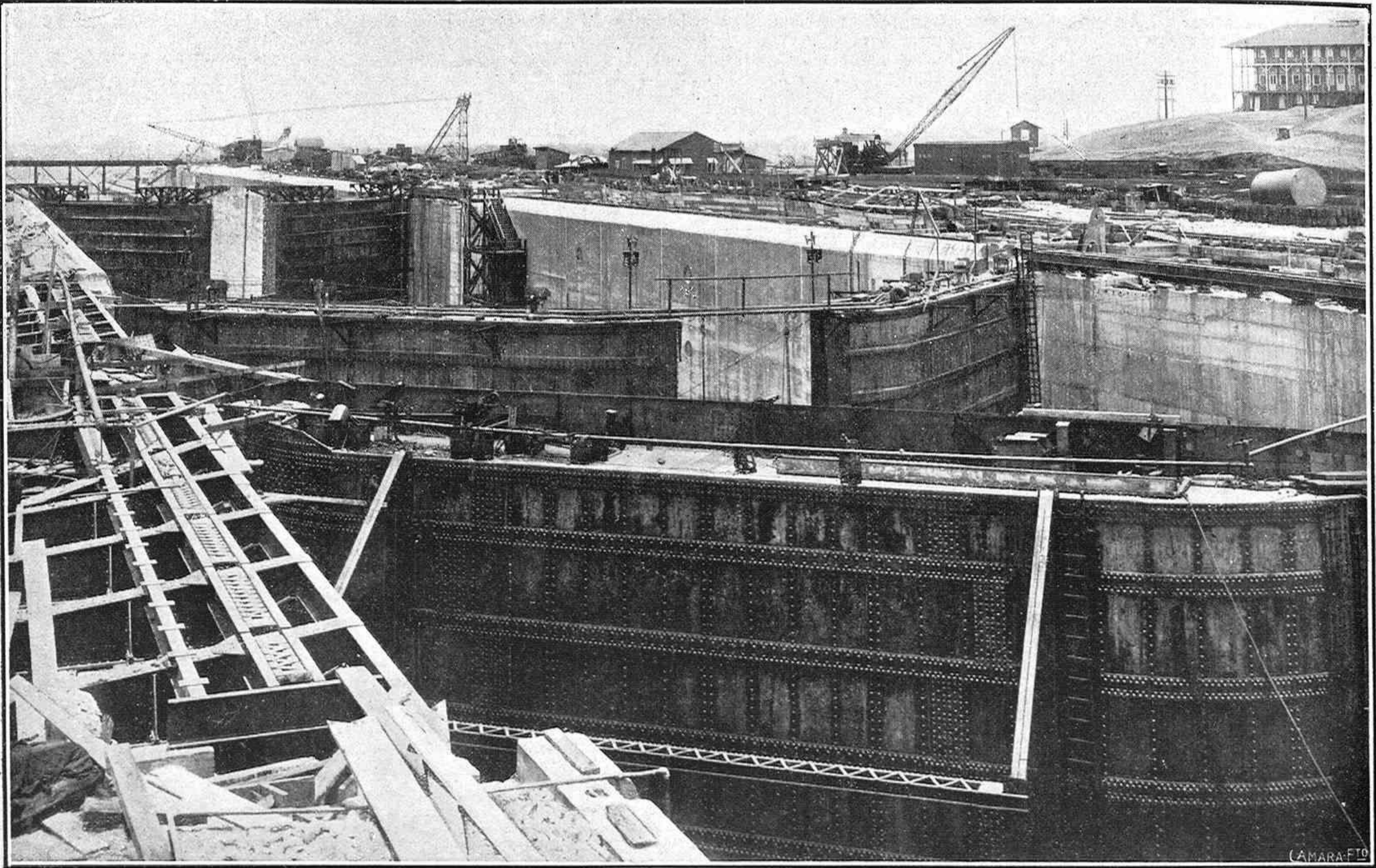
Construcción de un juego de compuertas en las esclusas de Gatun
