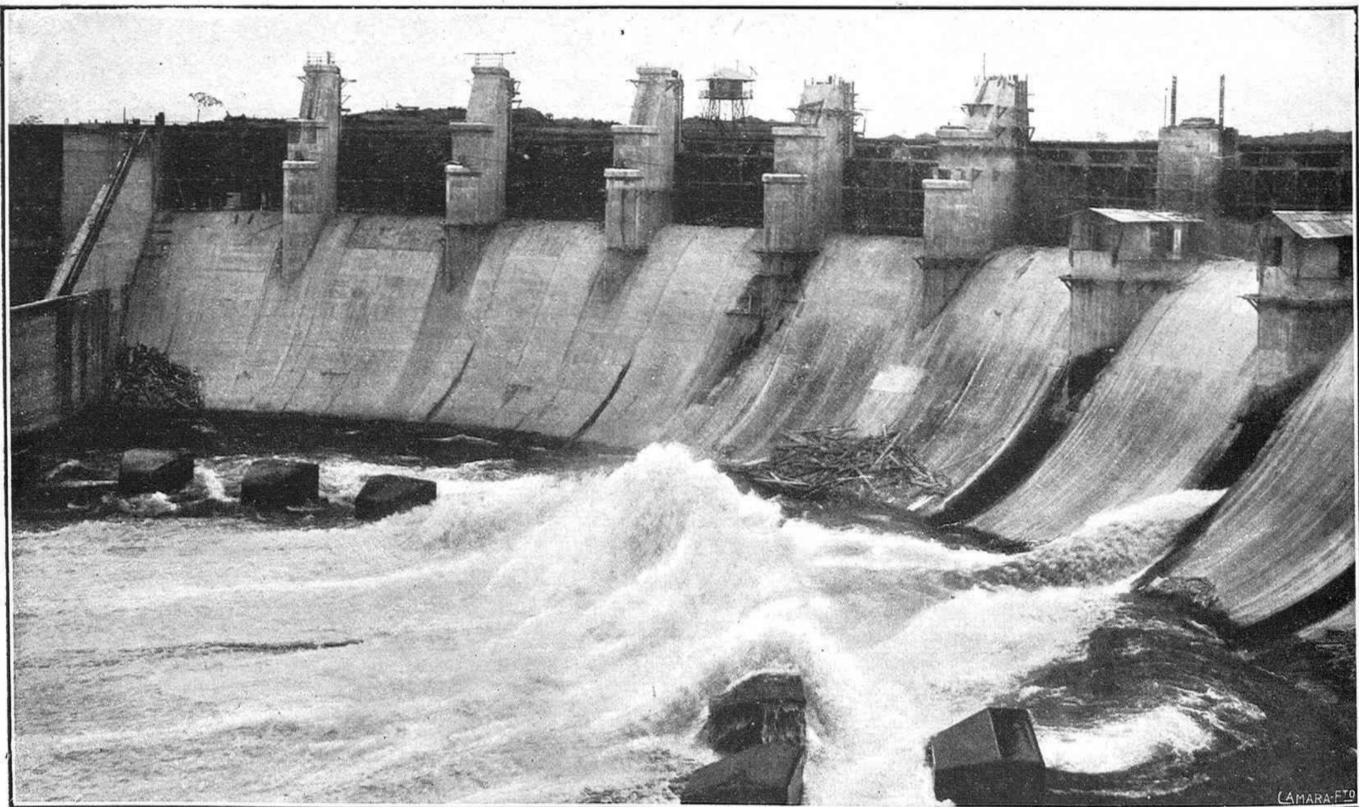
Uno de los desagües del lago de Gatun, que produce una energía de 5.000 caballos, aprovechados en el servicio del canal. La fotografía ha sido hecha antes de estar terminada la construcción del dique
