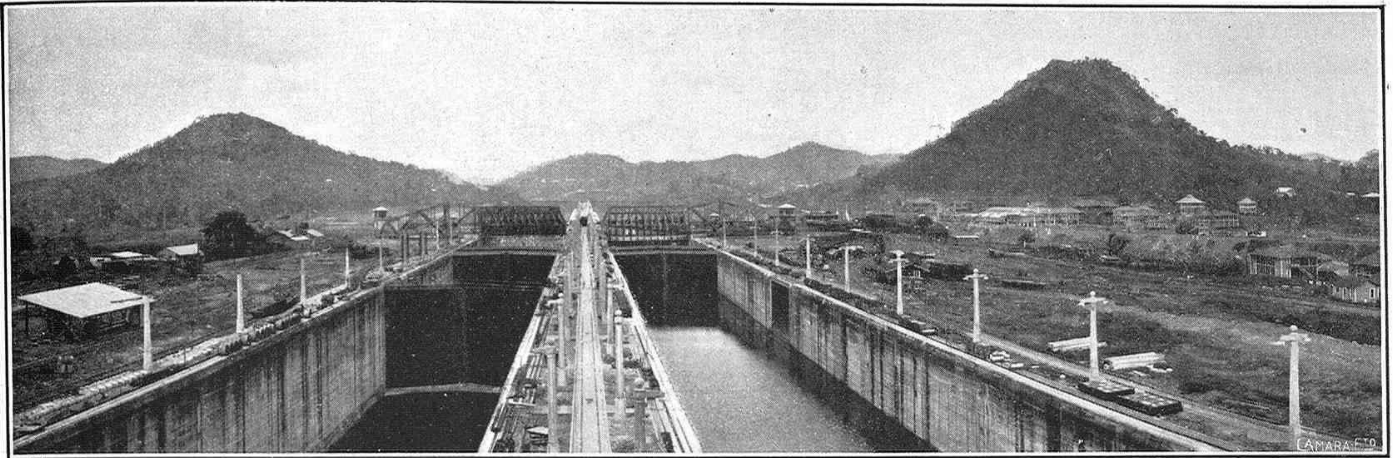
Esclusas de Pedro Miguel, mediante las cuales baja el nivel del lago de Gatun de 85 á 55 pies.—Al fondo se ven colocados los diques de emergencia
