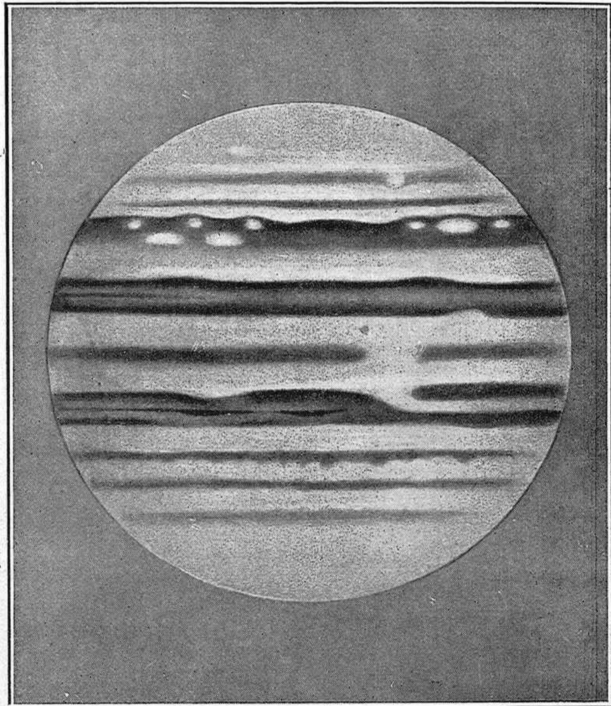
Aspecto del planeta Júpiter, que permite ver la uniforme y paralela distribución de sus bandas, las manchas brillantes en la región superior y un verdadero rosario de manchas oscuras en el hemisferio opuesto.—(Fotografía obtenida con la gran ecuatorial de Lick (California))
