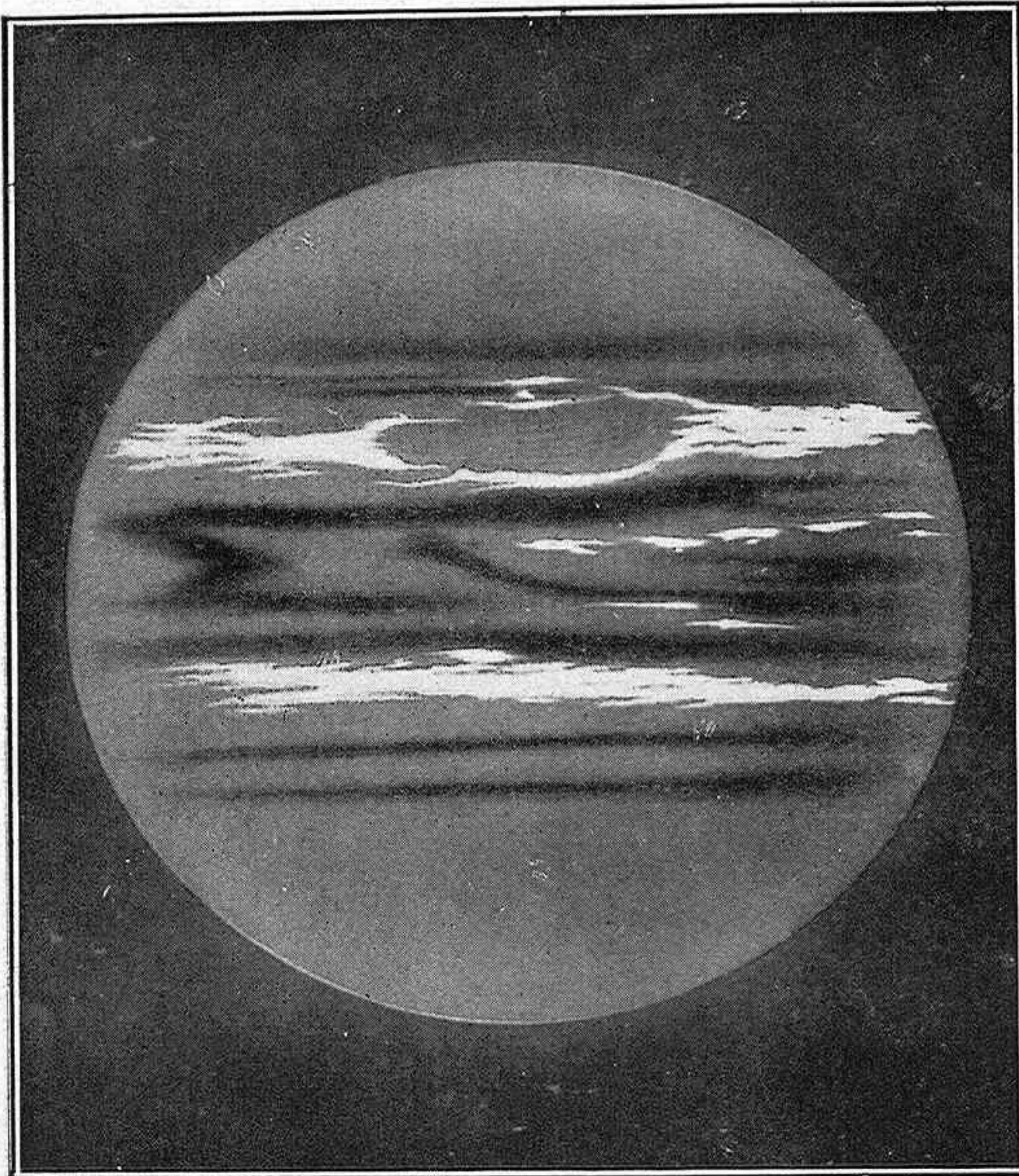
Curiosa disposición de las bandas de Júpiter, oscuras y brillantes, repartidas a uno y otro lado de su ecuador. En él, hacia la región media é izquierda del grabado, se ve la gran mancha, de fuerte coloración roja en la realidad.—(Fotografía obtenida con la gran ecuatorial del Monte Wilson (California))
