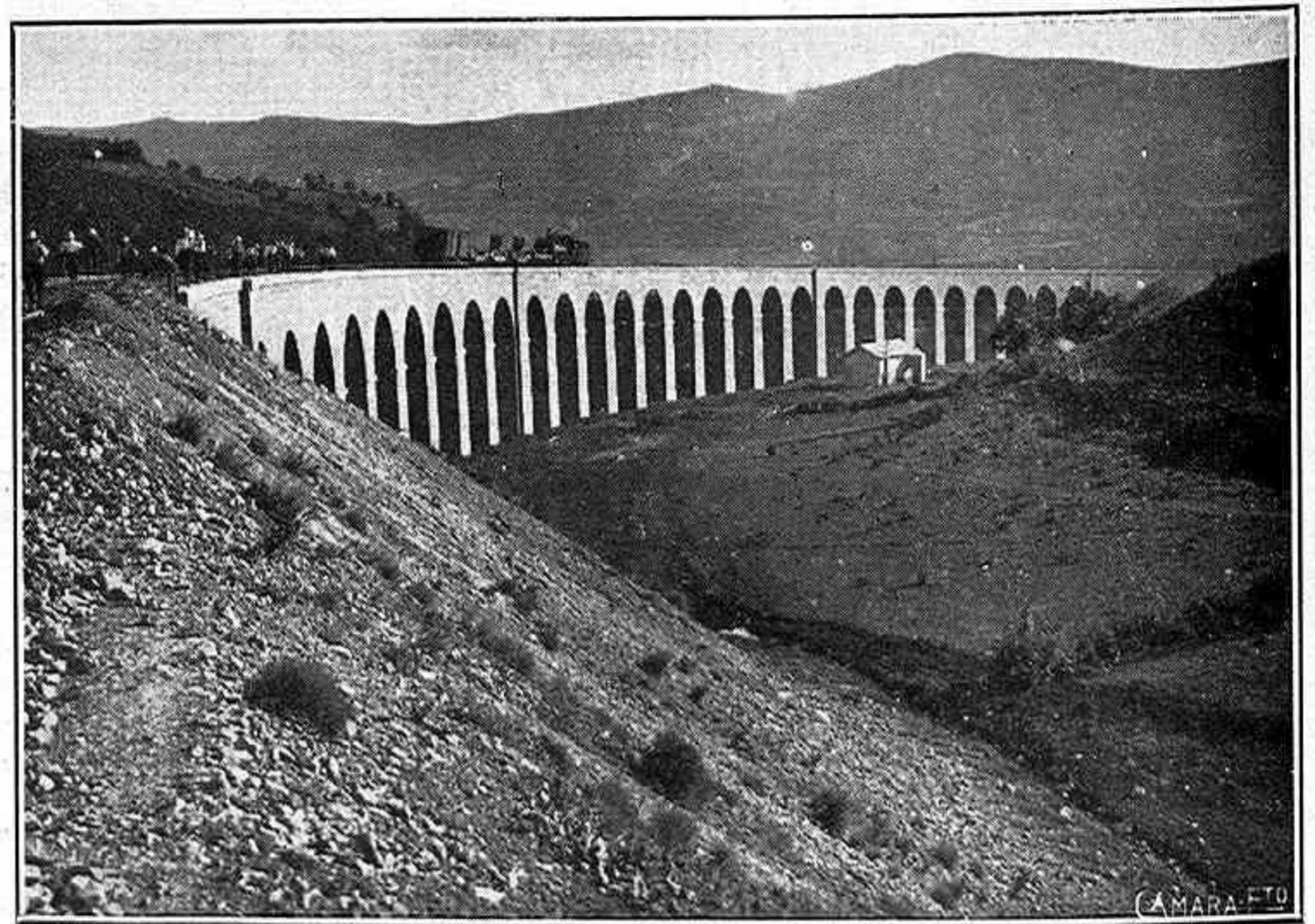
El magnífico viaducto de San Juan, que tiene veintiocho arcadas, diez y ocho metros de altura y treinta y cinco de longitud
