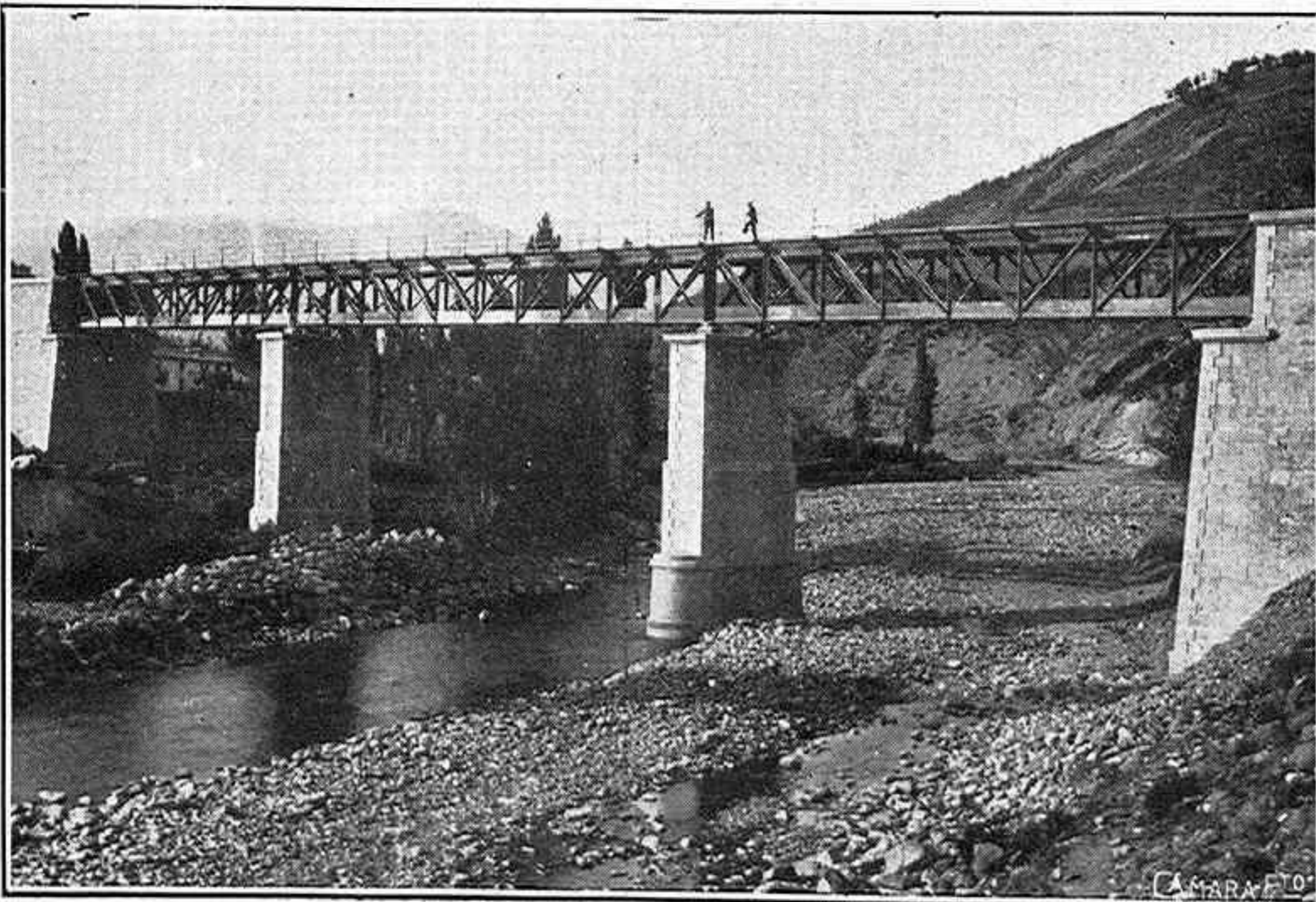
Puente de ochenta metros de longitud, construído para el paso del ferrocarril de Canfranc, sobre el río Aragón, en Castiello
