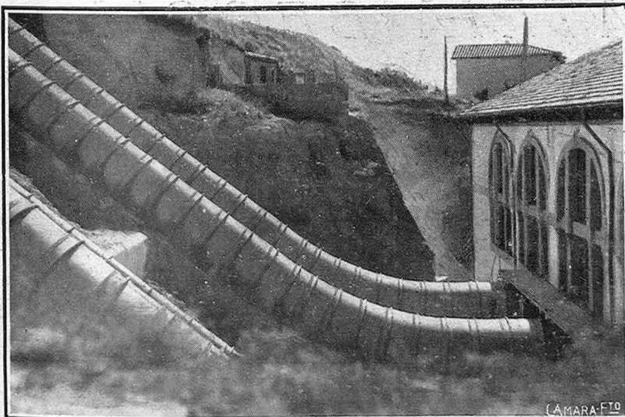
Las tuberías del salto
