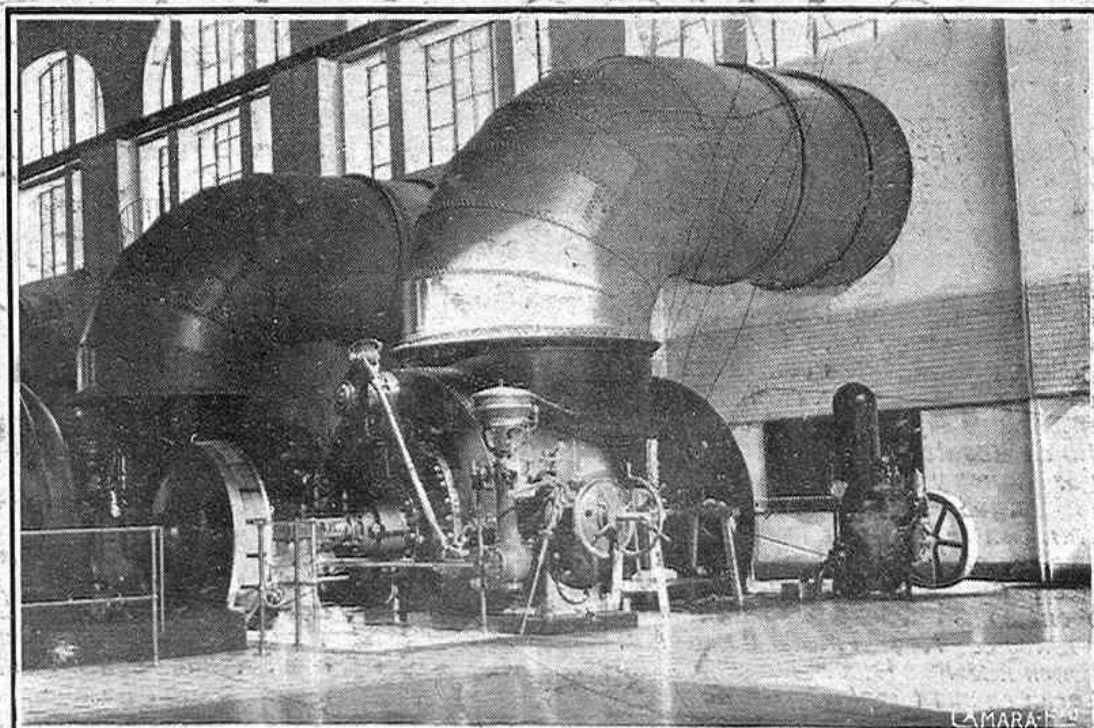
Detalle de la maquinaria
