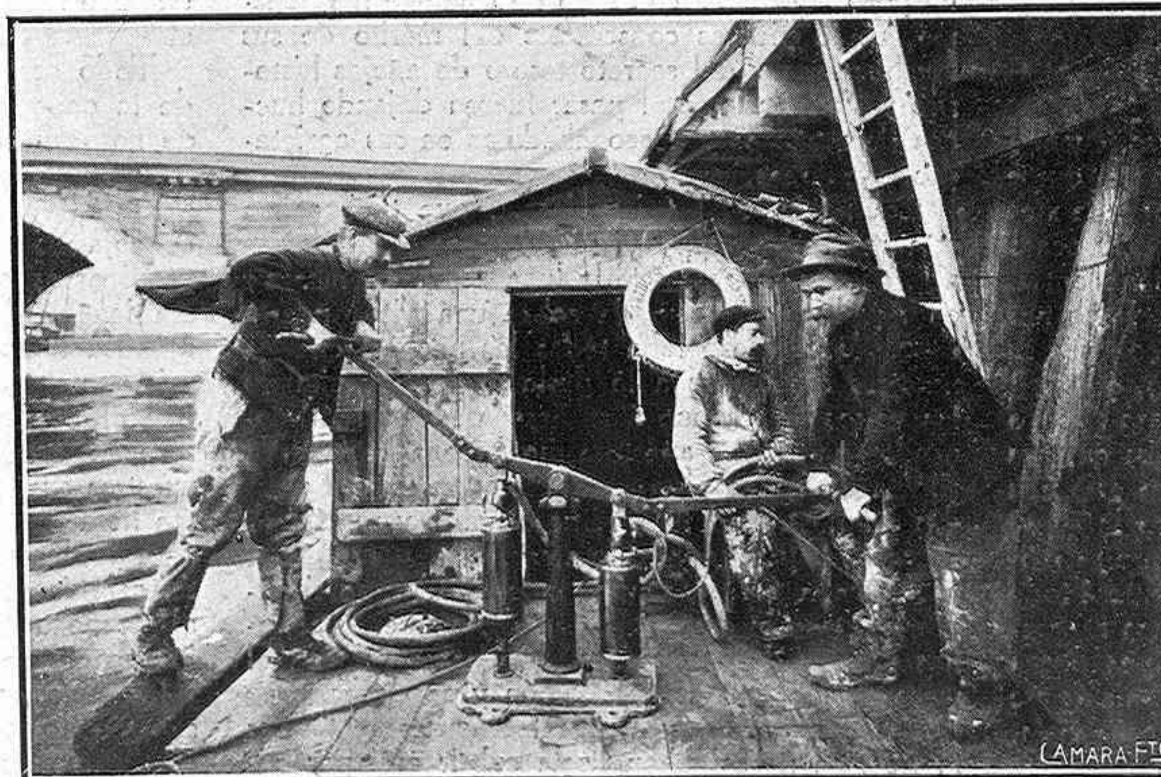
Bomba con la que se envía el aire al buzo durante sus operaciones en el fondo del mar FORS. BOYER
