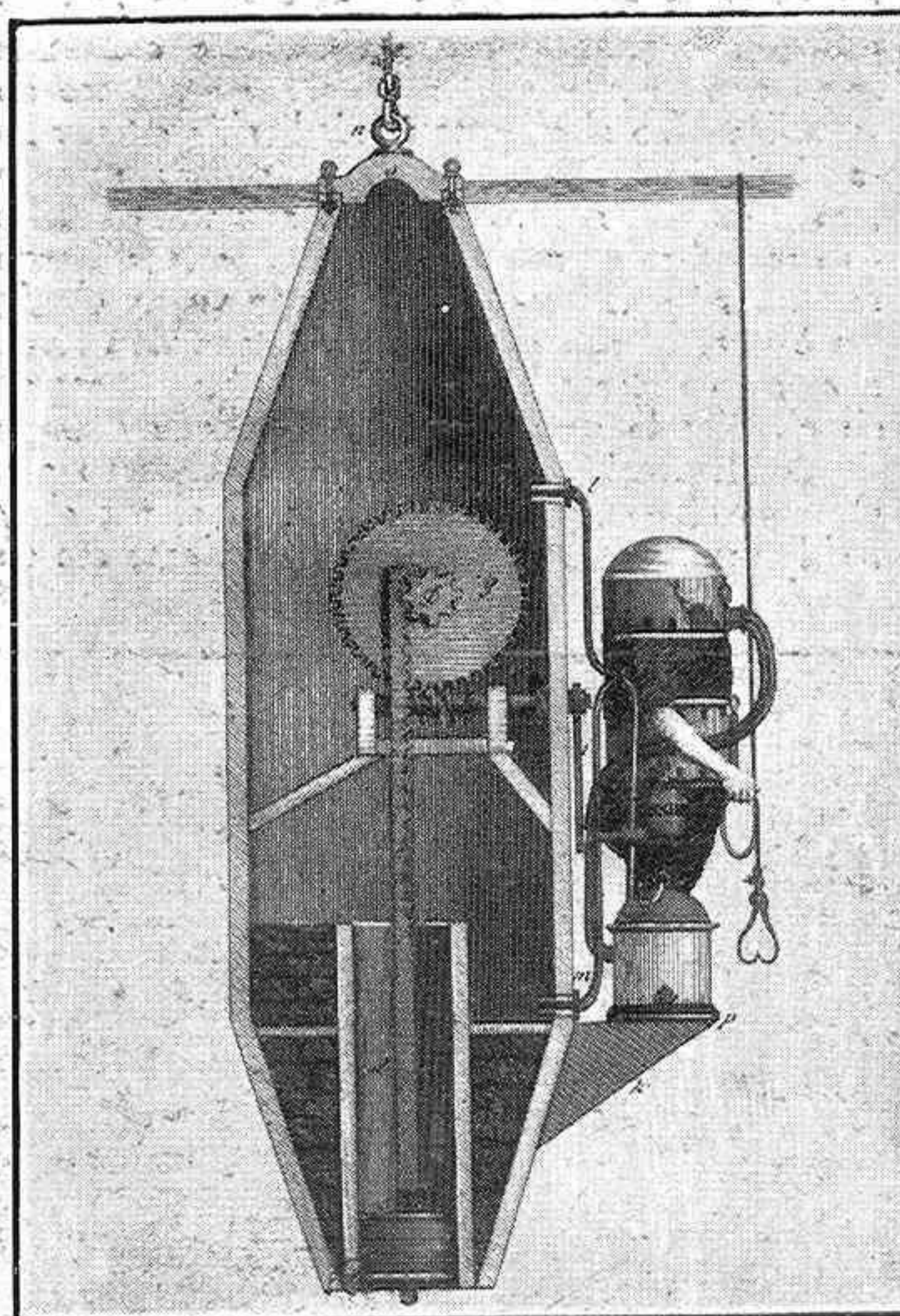
Conjunto del aparato Klingert para descender al fondo del mar
