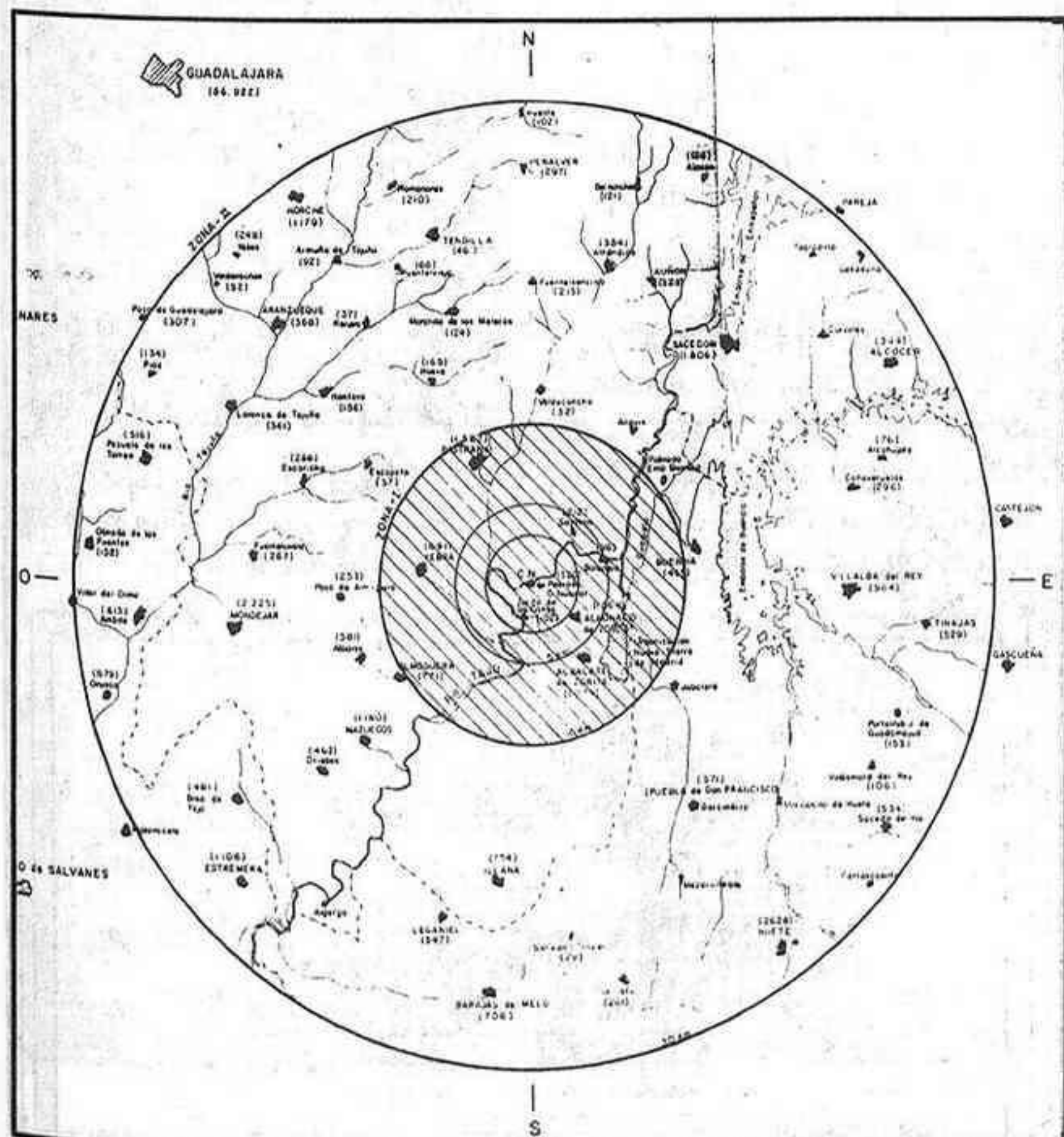
Area de 30 kilómetros Central de Zorita. La zona II del Plan de Emergencia Nuclear se corresponde con el último círculo concéntrico.
