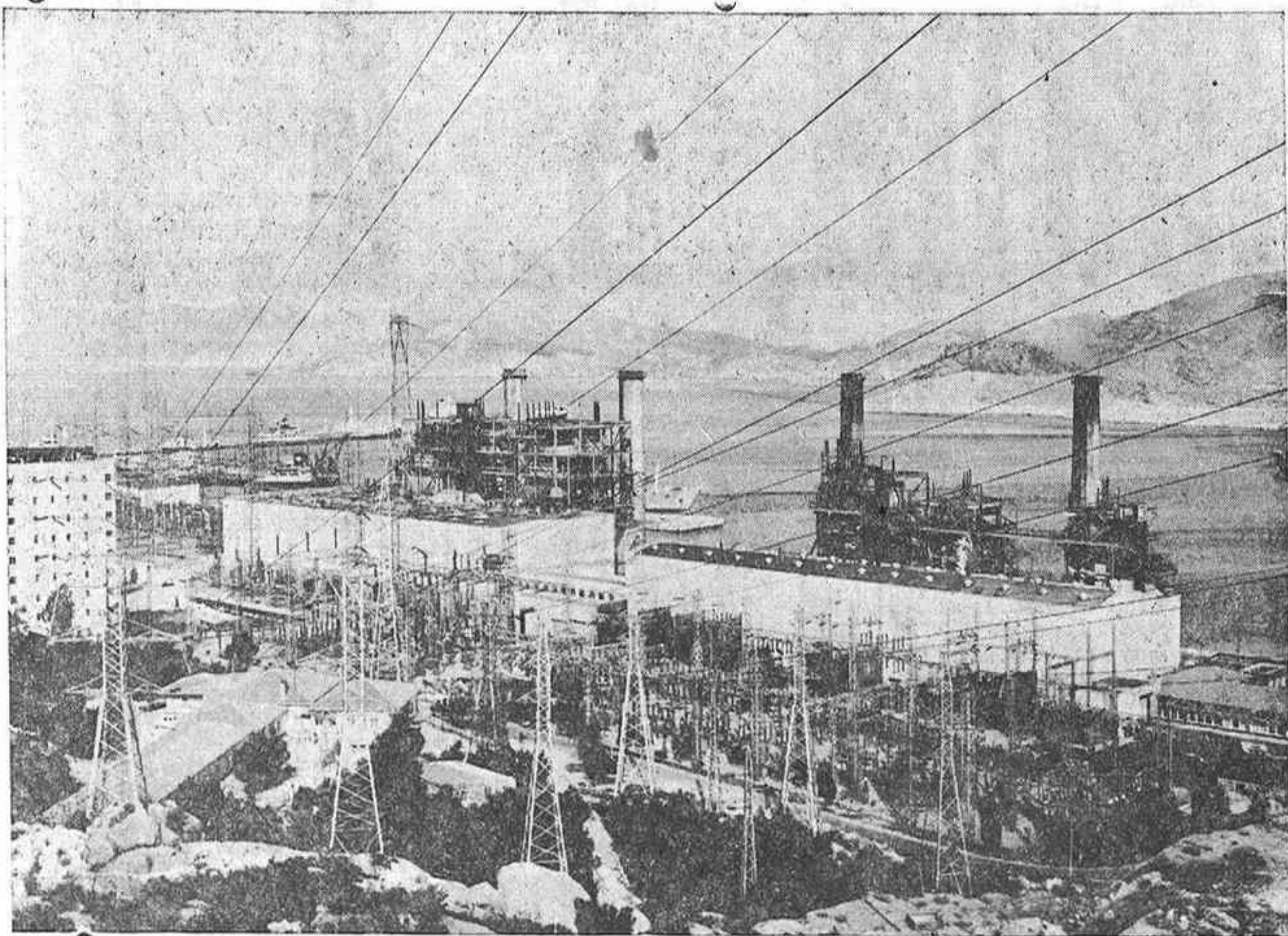
Complejo térmico de Escobrerías (Murcia). Potencia: 858.000 kw. Producción anual. 6.500 millones de kwh.
