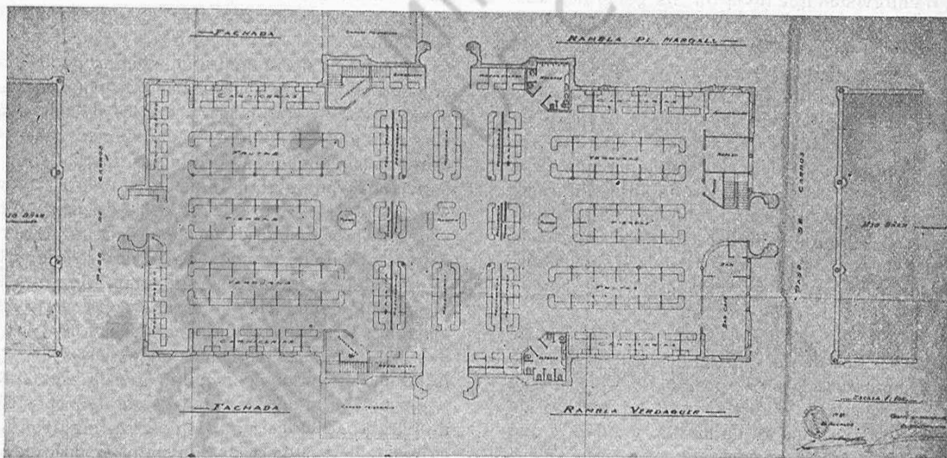
Distribución de la Planta de la Plaza Mercado
