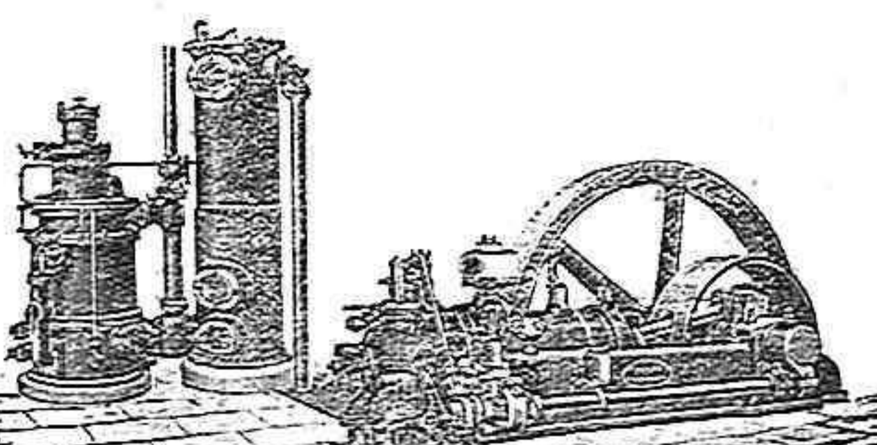
Motor de gas pobre con gasógeno.
