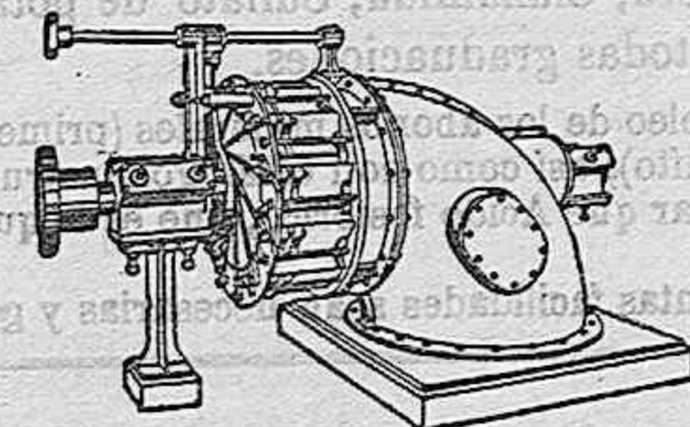
Turbina horizontal "Simsom".
