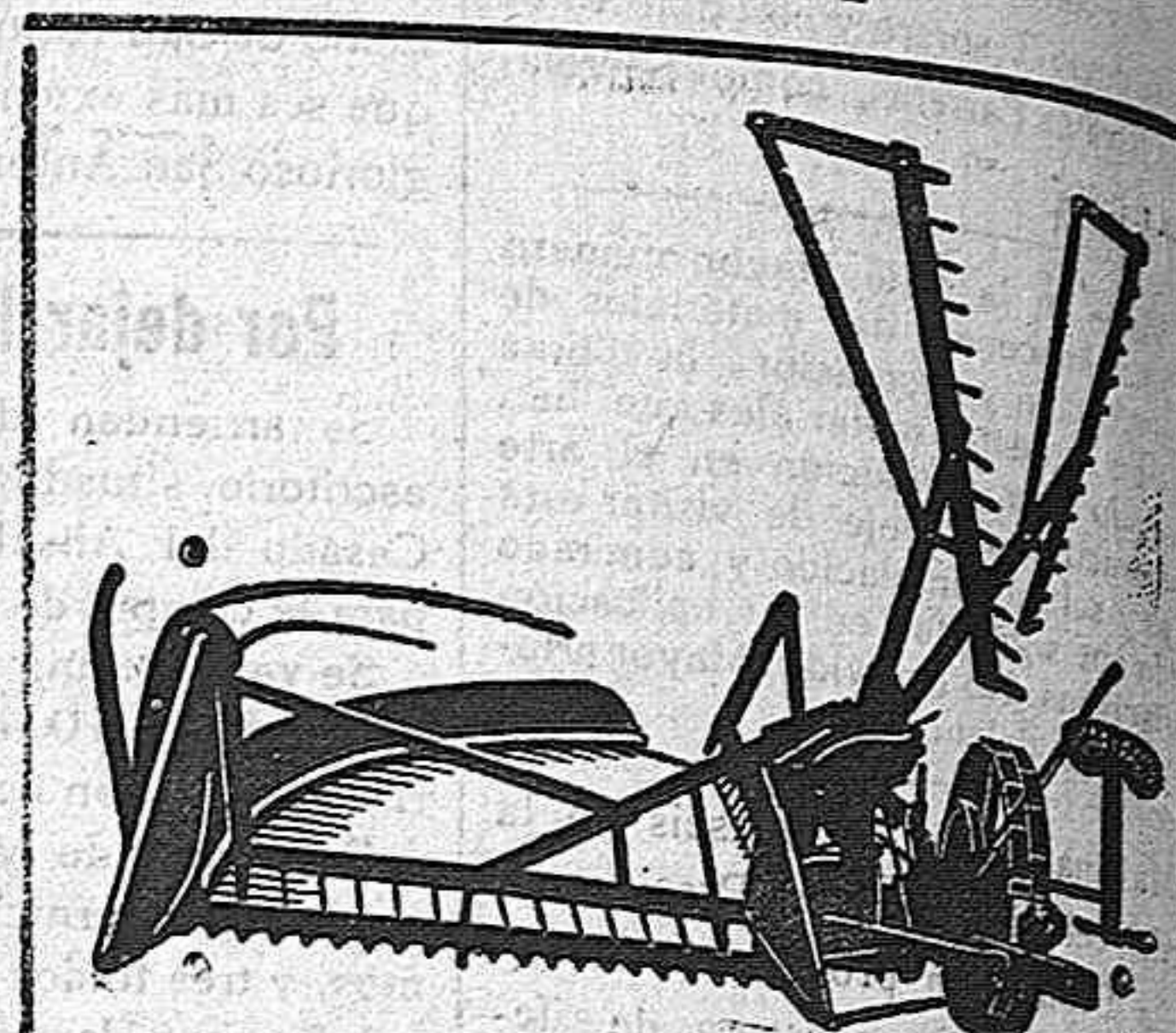
Agavilladora de 1 1/2 metros de corte para un par corriente
