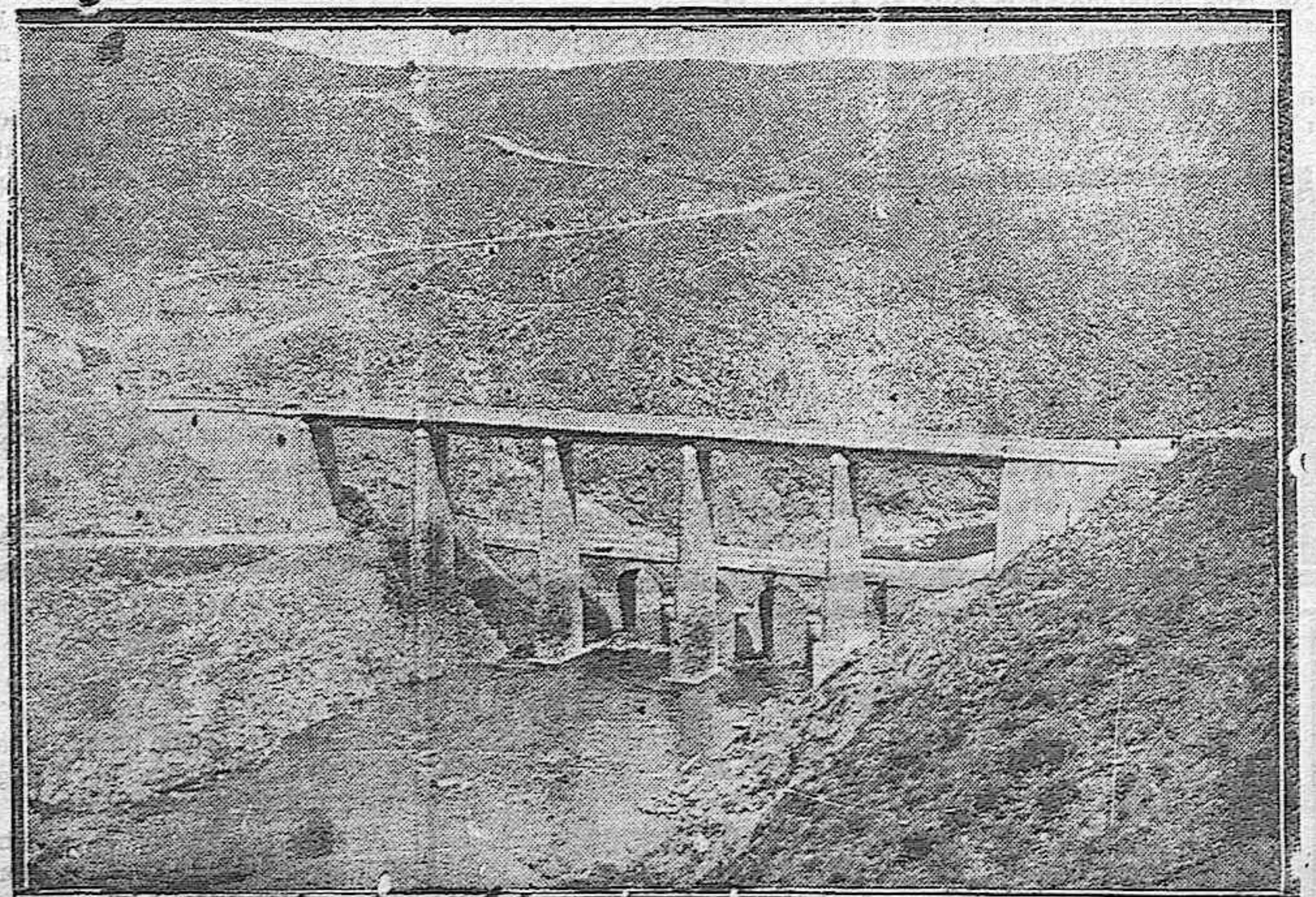
LAS OBRAS DE LA CONFEDERACION DEL DUERO.—Nuevo puente en el río Agueda en la zona del embalse del pantano de su nombre.
