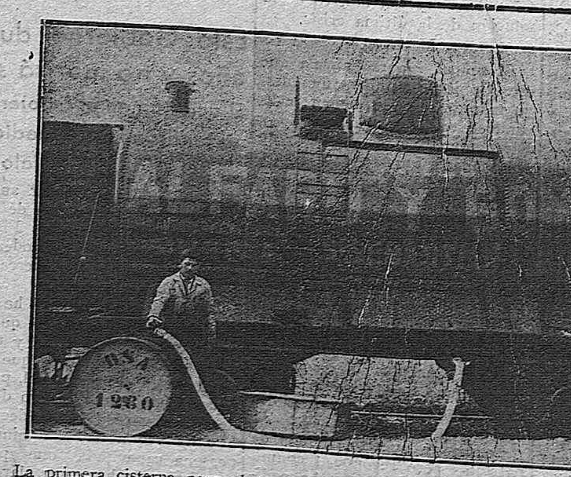
La primera cisterna para el transporte de aceites recibida en Palencia. Fué consignada a los Almacenes de Alejandro Ortega, y tiene de capacidad 10,966 kilos, transportando un finísimo aceite que beneficia enseguida de la ventaja de un transporte económico, de máxima limpieza y seguridad, por ningún otro envase.
