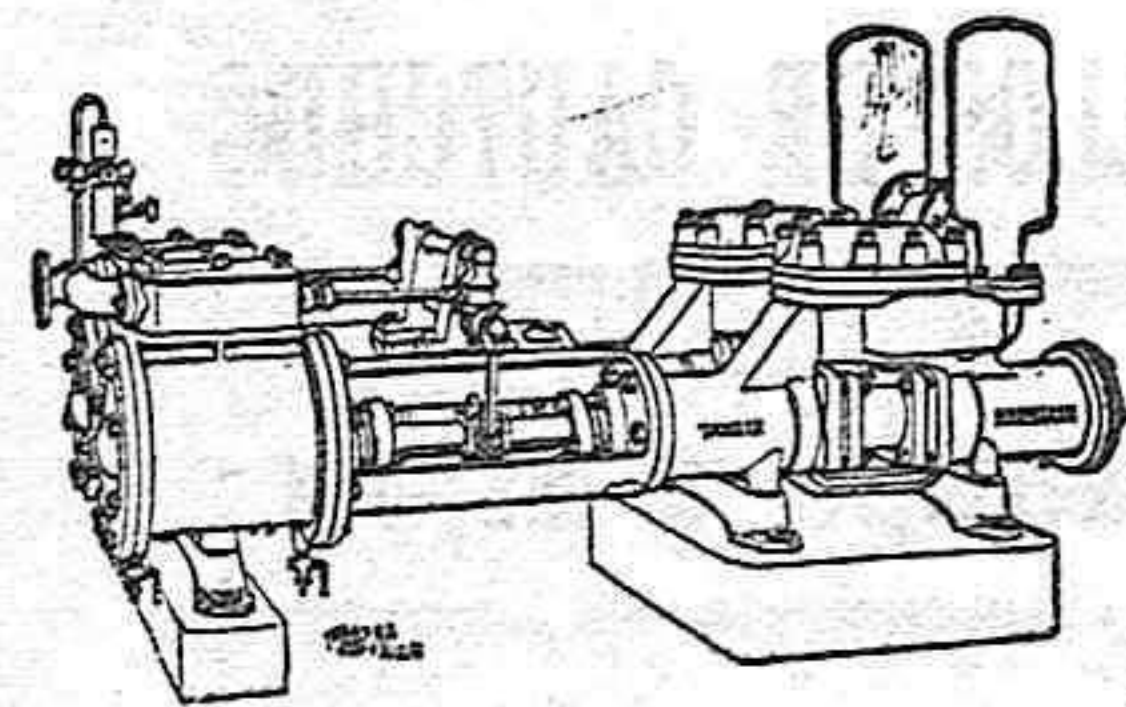
Bomba «Tangyes»
