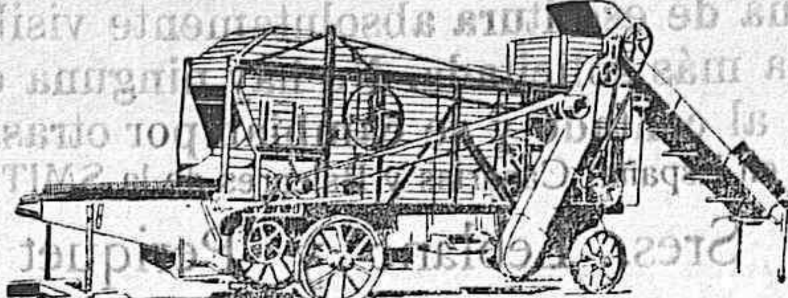
Trilladora «Triunfo Grande» con elevador de mies. Rendimiento diario de 150 a 200 fanegas de trigo, según granazón.
