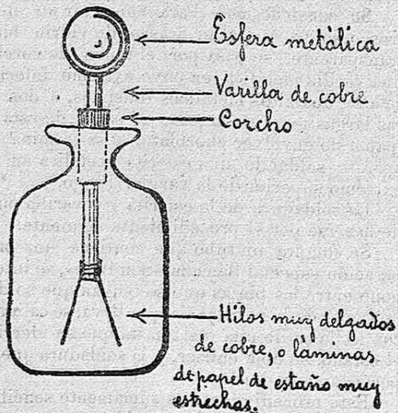
Fig. 5 — Electroscopio
