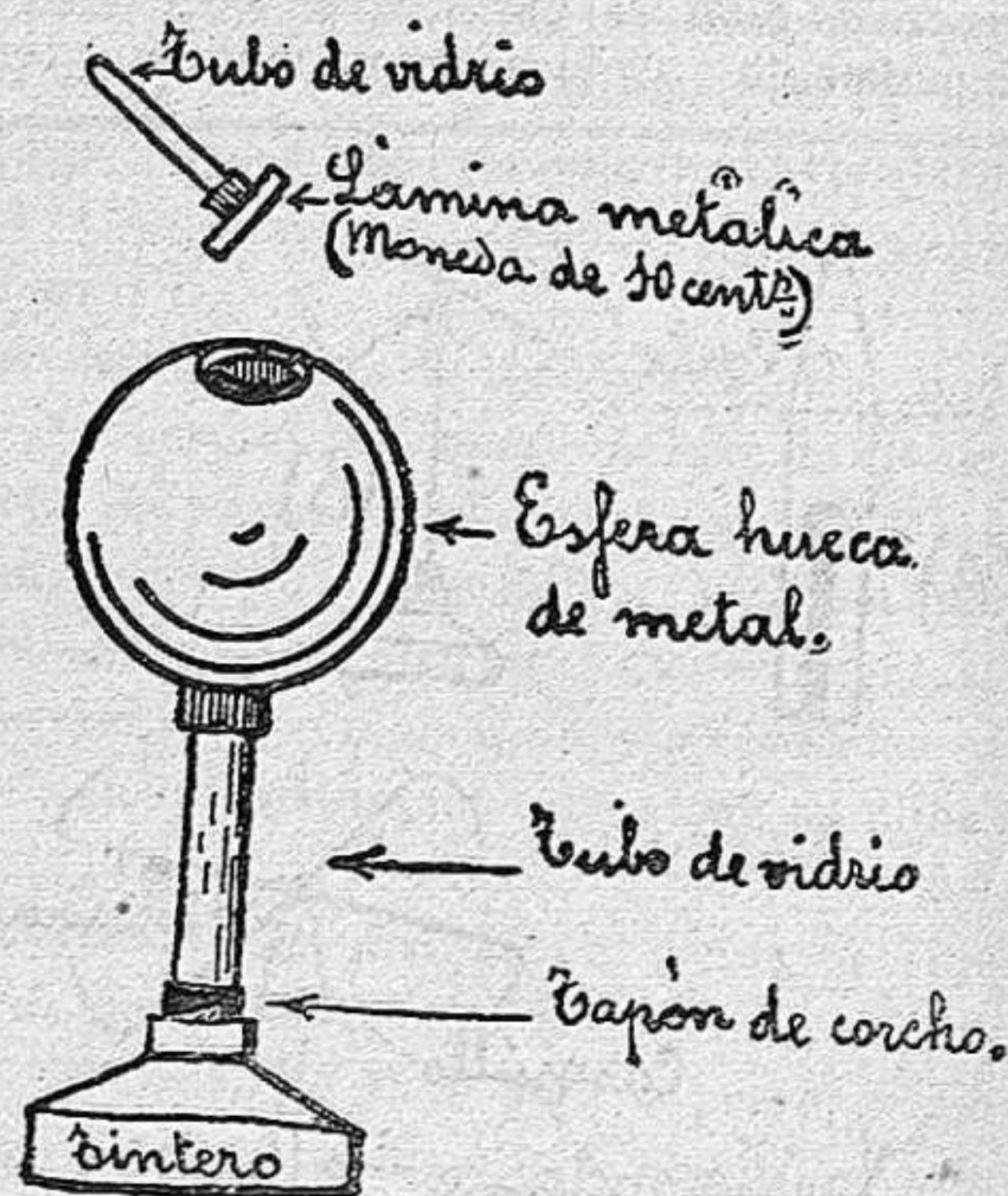
Fig. 6.—Esfera de Coulomb
