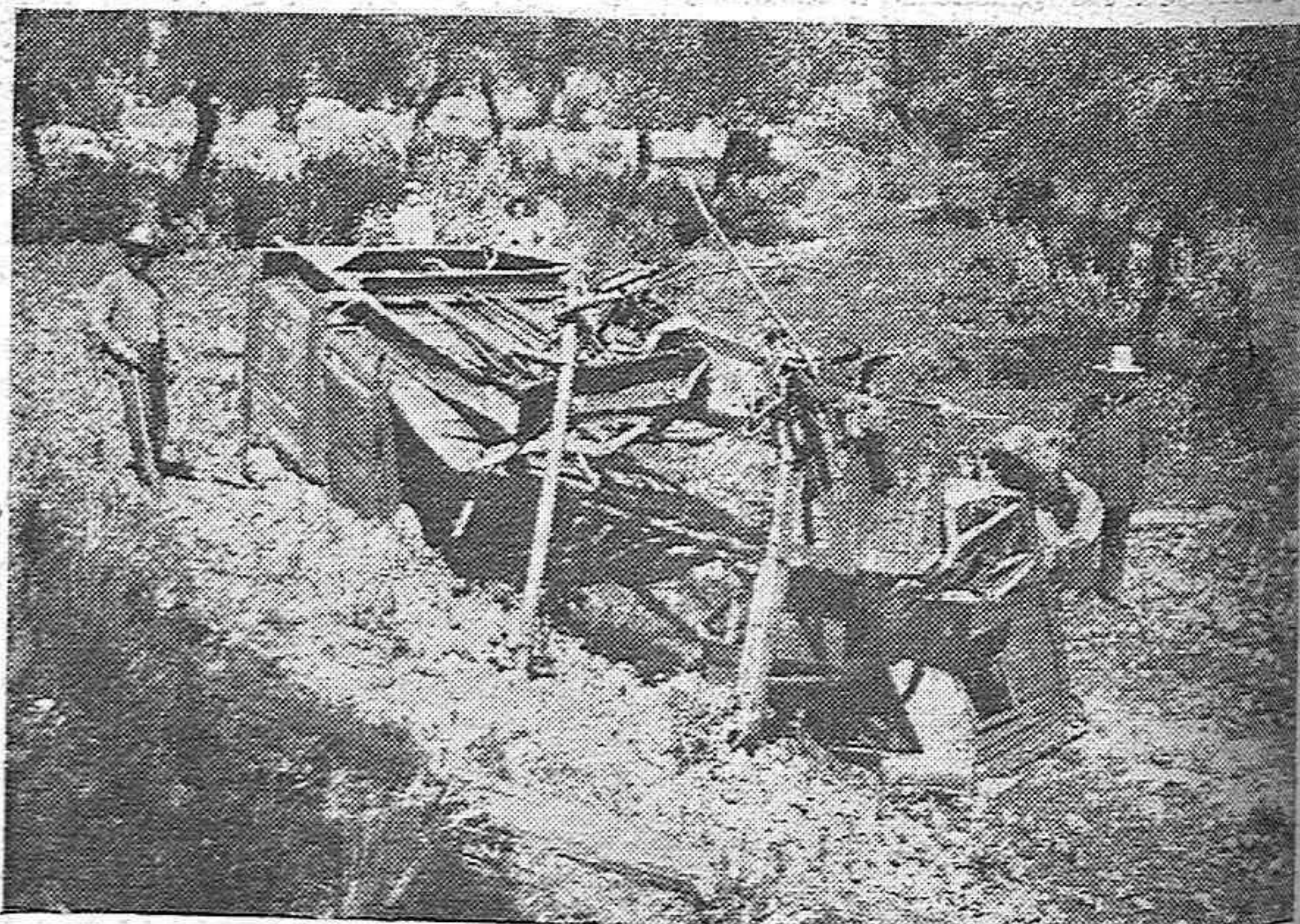
EL DESCARRILO DE AYER EN LA LINEA DE LA SIERRA. —ESTADO EN QUE QUEDÓ PARTE DEL CONVOY AL DESPEÑARSE UNOS VAGONES POR UN TERRAPLEN DE BASTANTE ALTURA.
